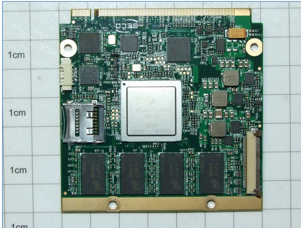
CPU module SECO Q928-V5C0 - Top
