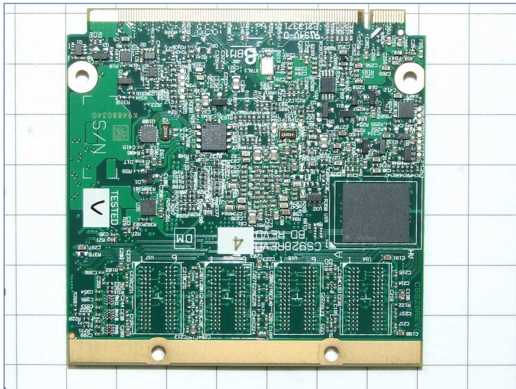
CPU module SECO Q928-V5C0 - Bottom
