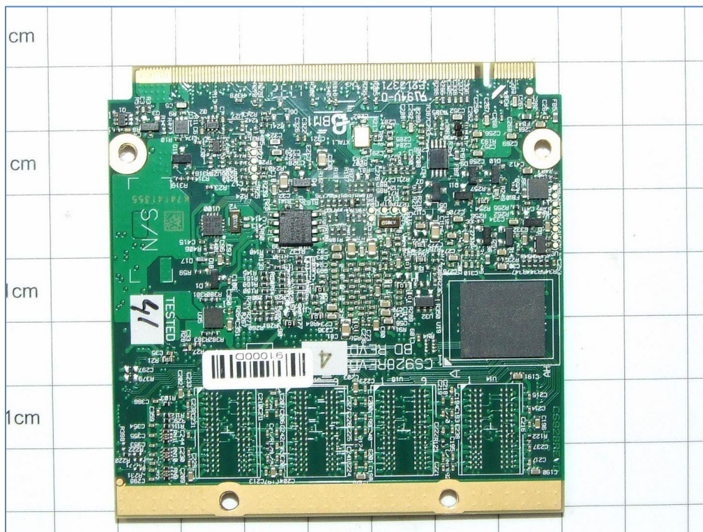
CPU module SECO Q928-V3C0 - Bottom
