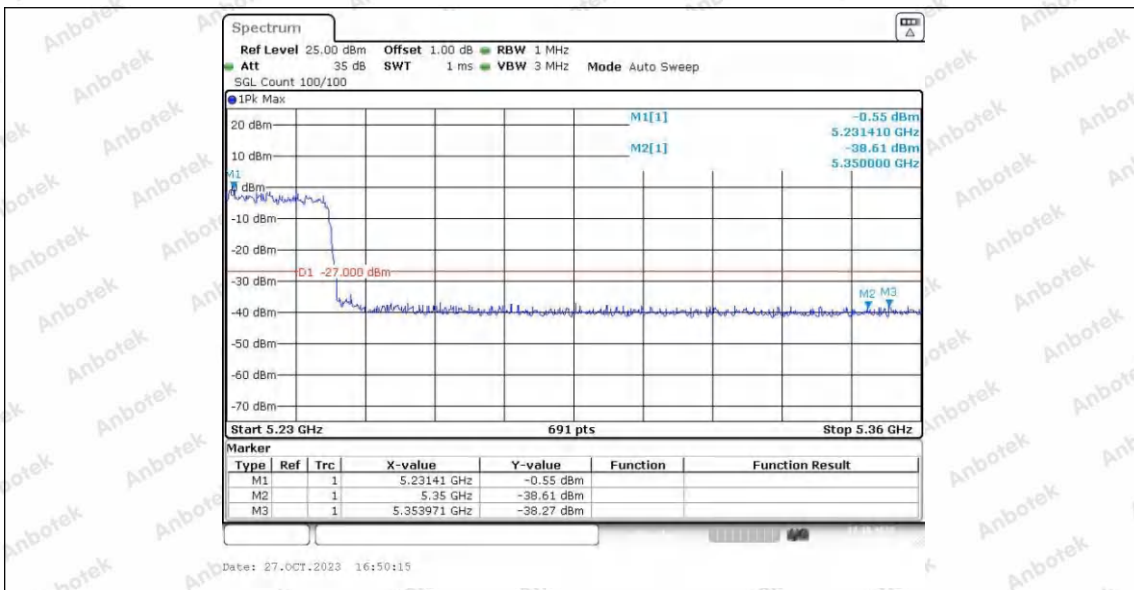
11AX80SISO_Ant1_Low_5290
