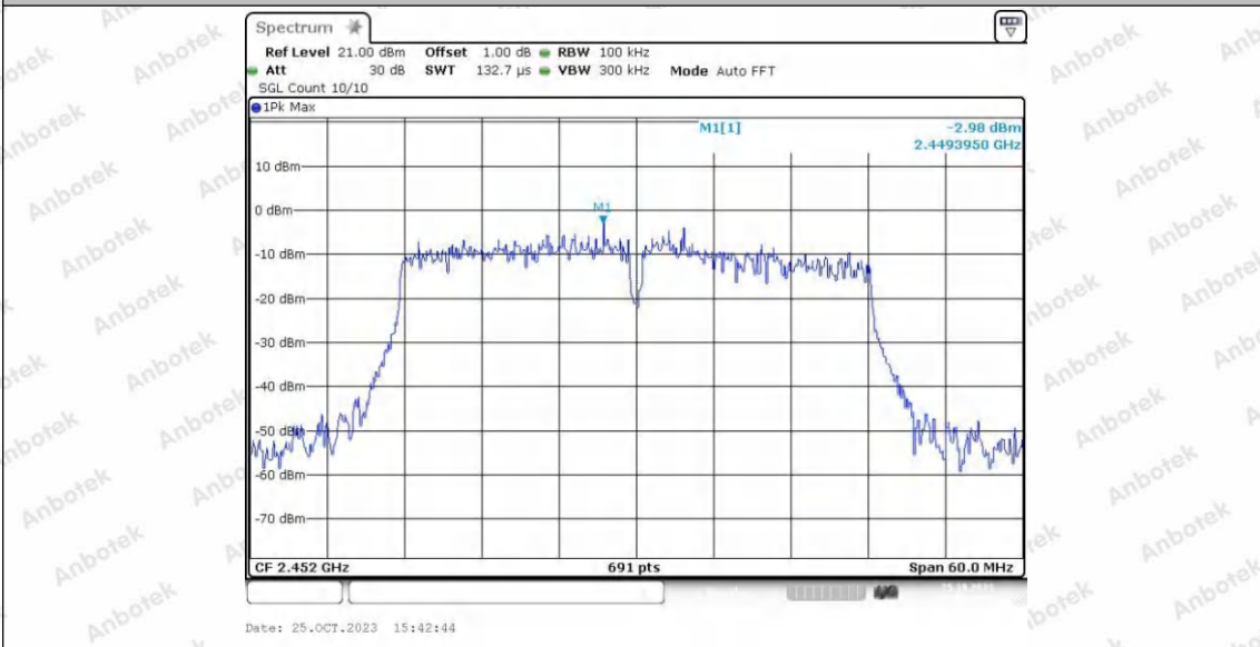
11N40SISO_Ant2_2452_30~100
