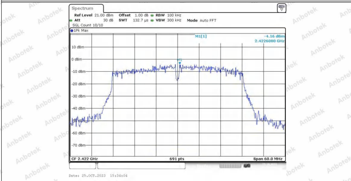
11N40SISO_Ant2_2422_30~100
