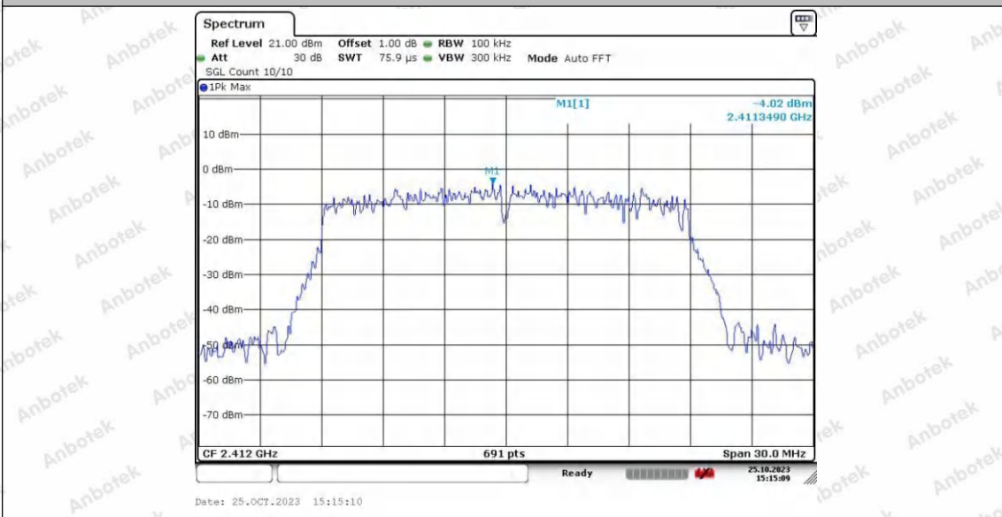
11N20SISO_Ant2_2412_30~100
