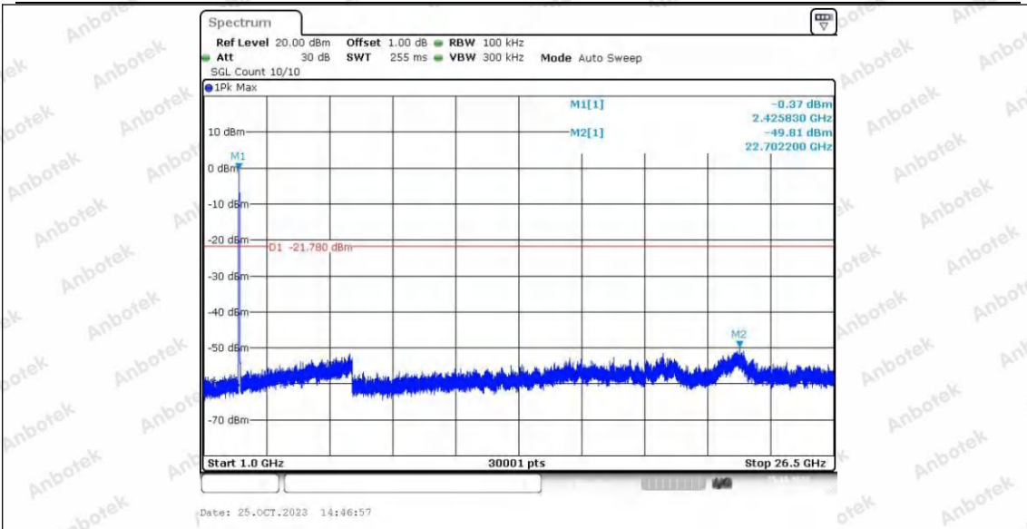
11AX40SISO_Ant2_2422_0~Reference
