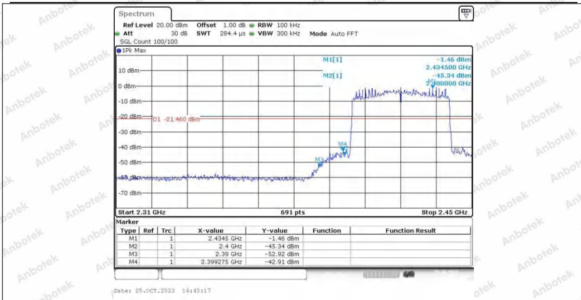
11AX40SISO_Ant2_Low_2422
