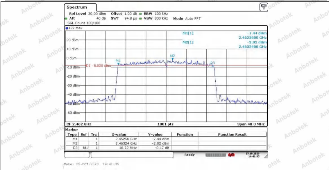
11AX20SISO_Ant2_2462
