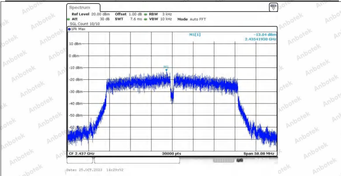
11N40SISO_Ant2_2437
