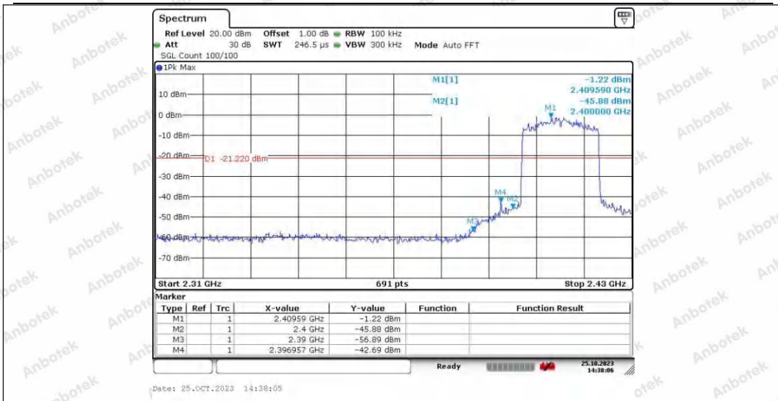
11AX20SISO_Ant2_Low_2412
