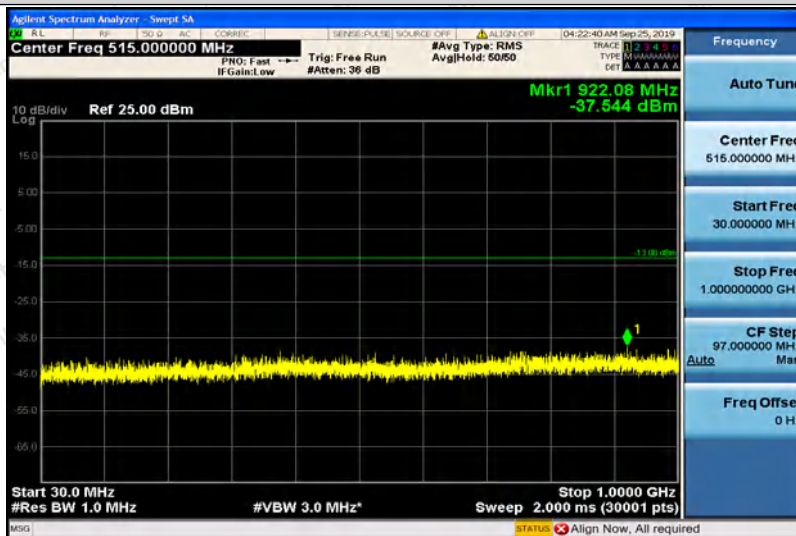
Band2-10MHz-16QAM-18900-1RB#0-Range2:1000~5000MHz
