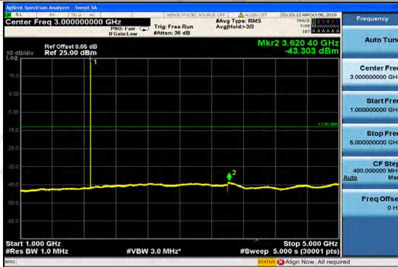
GPRS1900-661-1000~5000
