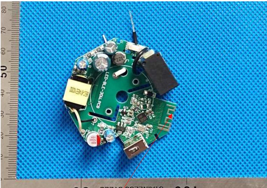
antenna.
