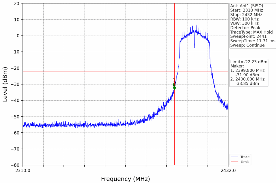
802.11n(HT20)_LCH_2412MHz_Ant1 (SISO)_NTNV
