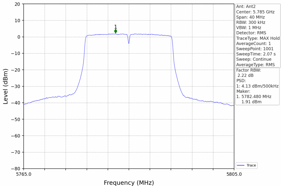
802.11a_MCH_5785MHz_Ant2_NTNV
