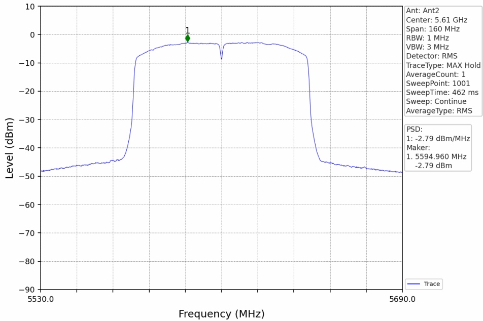
802.11ac(VHT80)_HCH_5610MHz_MIMO_NTNV
