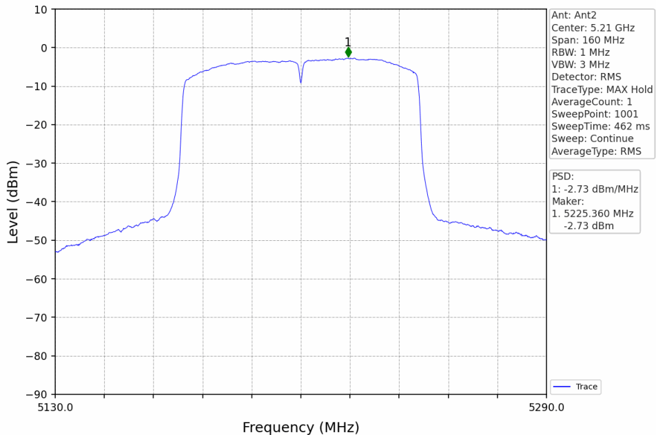
802.11ac(VHT80)_MCH_5210MHz_Ant2_NTNV
