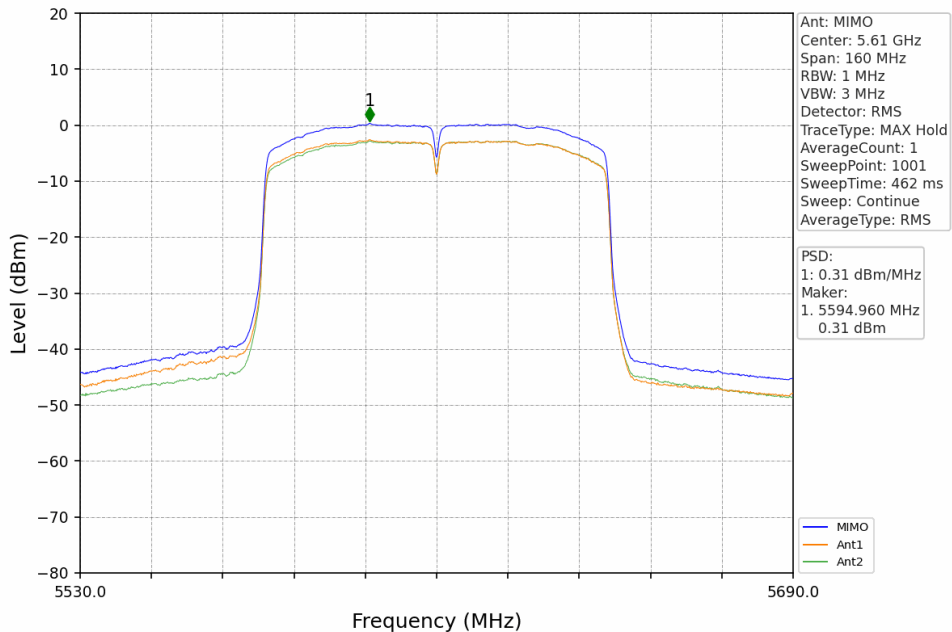
802.11ac(VHT80)_HCH_5610MHz_MIMO_NTNV
