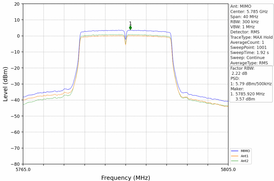
802.11n(HT20)_MCH_5785MHz_MIMO_NTNV
