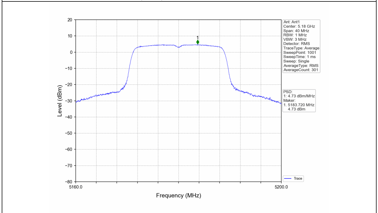
802.11n(HT20)_LCH_5180MHz_Ant1_NTNV
