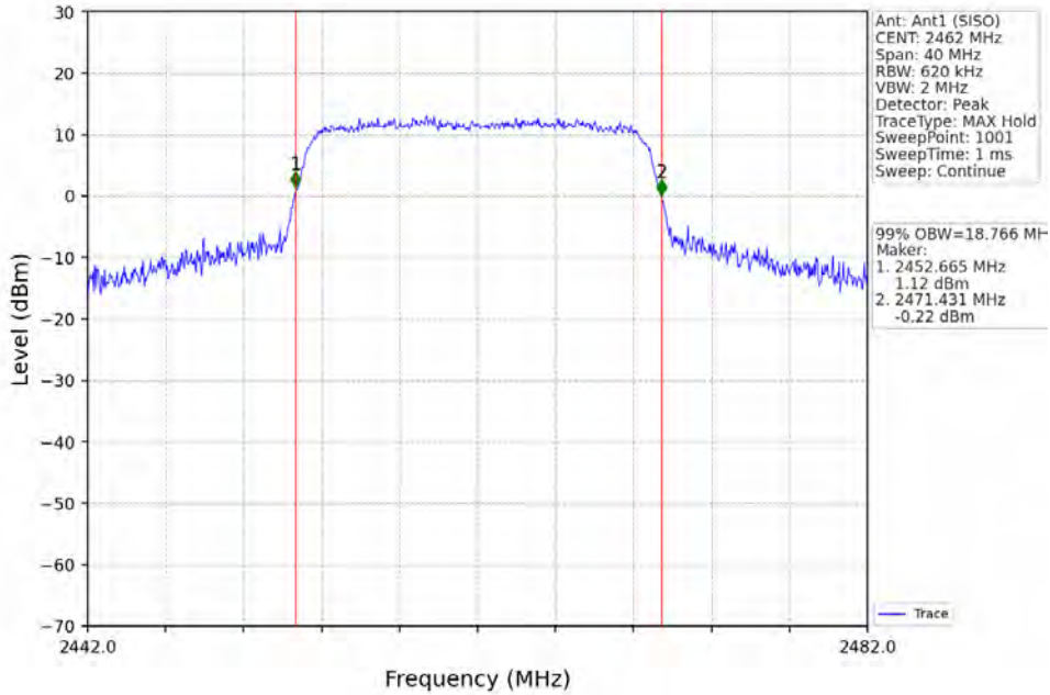
802.11n(HT20)_HCH_2462MHz_Ant1 (SISO)_NTNV
