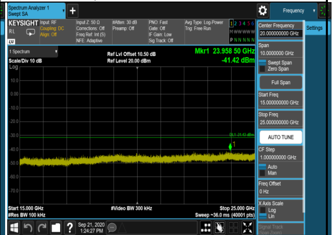
802.11n(HT20),2462MHz,Ant0,Plot 6,15000MHz~25000MHz
