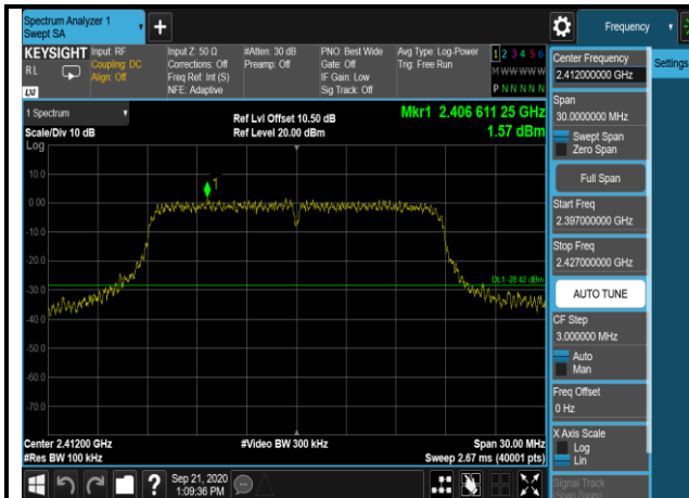
802.11n(HT20),2412MHz,Ant0,Plot 3,30MHz~2310MHz
