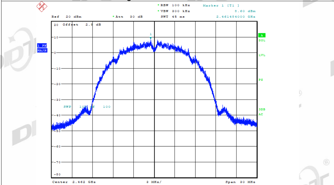
Band Edge NVNT b 2462MHz Ant1 Ref
