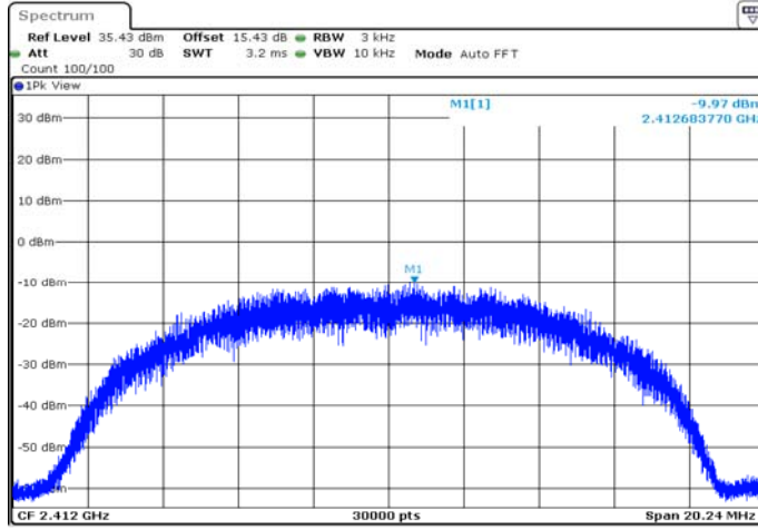
11B_Ant1_2412
