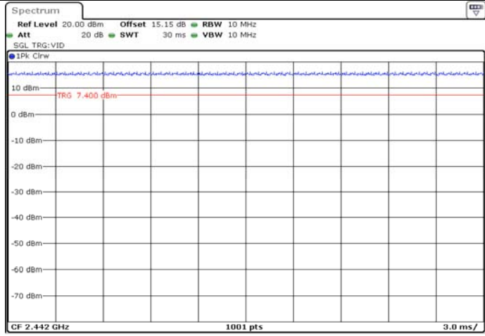
11N20_Ant1_2442
