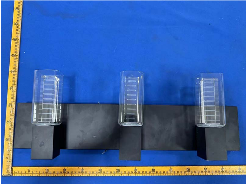
Fig.1(Model: VAN3-HOL5C )
