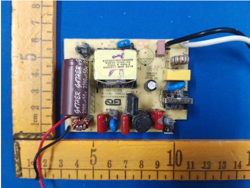
Fig.5(Model: OPDT-OPC)
