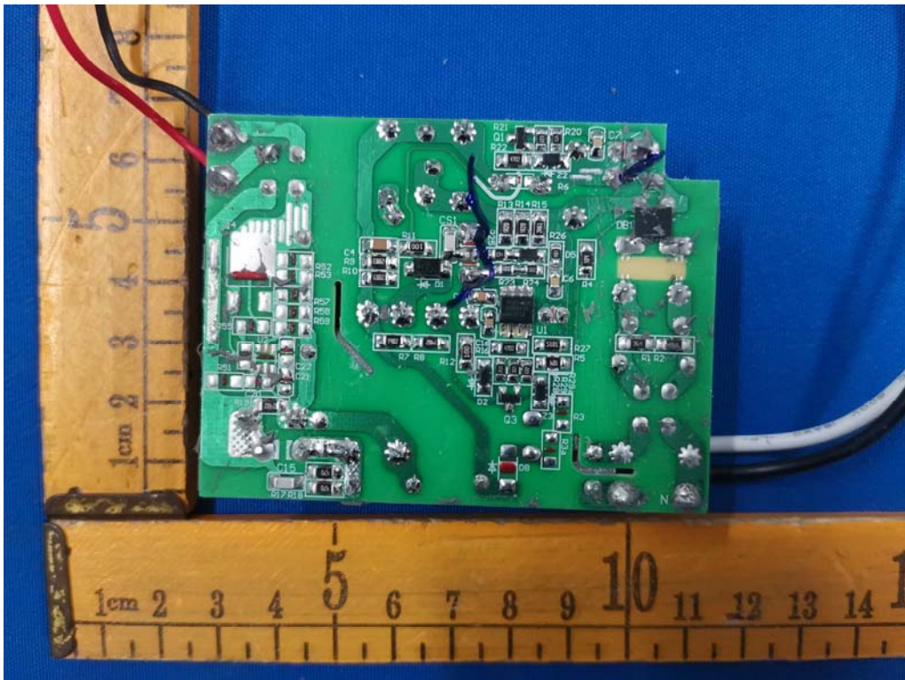
Fig.6(Model: OPDT-OPC)
