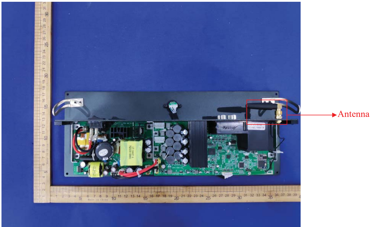
2) EUT Photo
