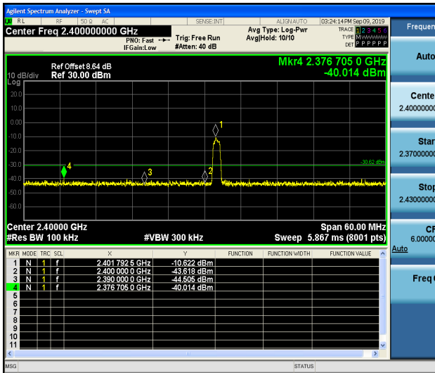
Left Band edge hopping off
