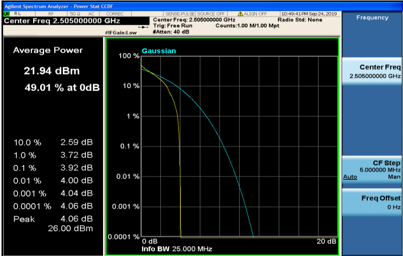
Band7-10MHz-QPSK-20800-50RB#0
