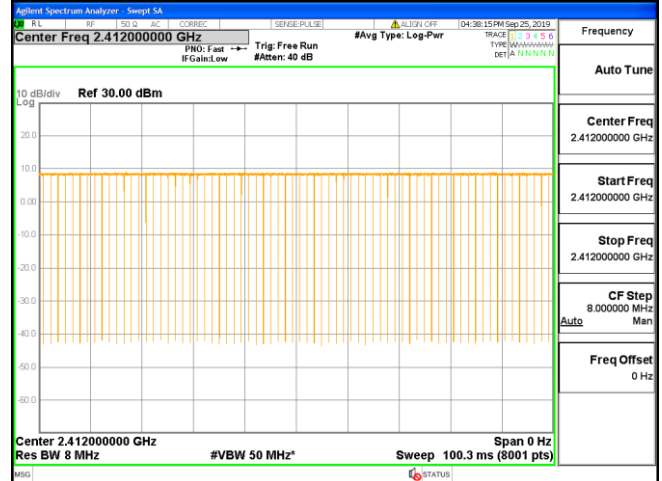
IEEE 802.11g
