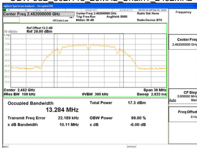
OBW 6dB 802.11b 20MHz Chain1 2462MHz
