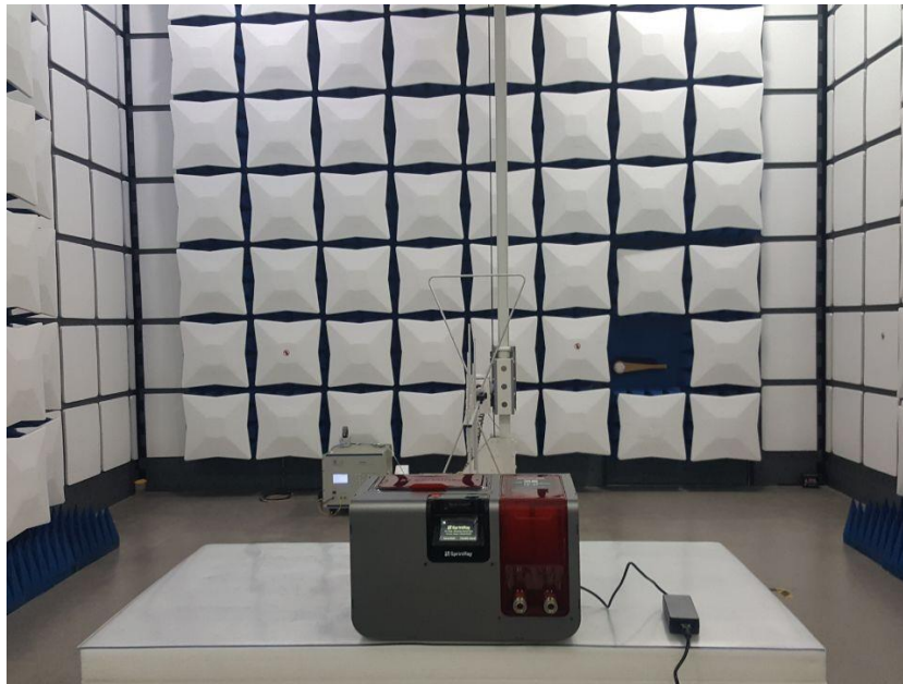
30MHz-1000MHz
