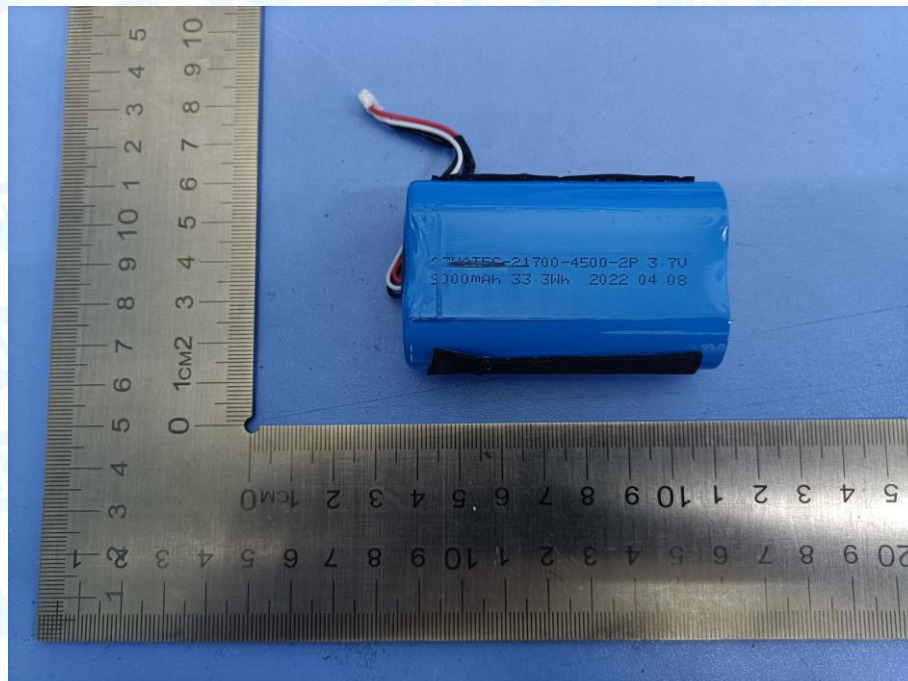
Photo 9 Battery parameters
