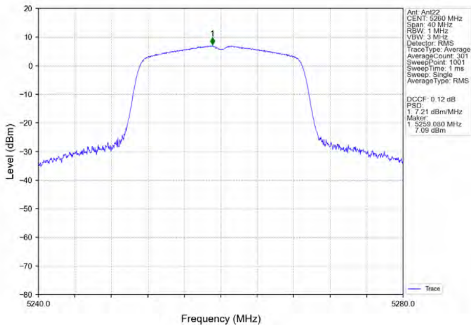
802.11n(HT20)_LCH_5260MHz_Ant22_NTNV
