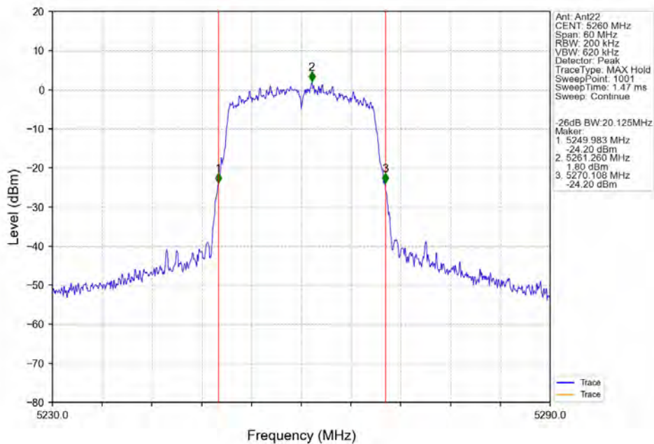
802.11n(HT20)_LCH_5260MHz_Ant22_NTNV
