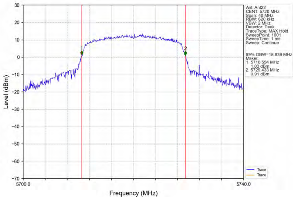
802.11n(HT20)_HCH_5720MHz_Ant22_NTNV
