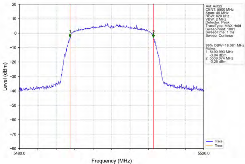
802.11n(HT20)_LCH_5500MHz_Ant22_NTNV
