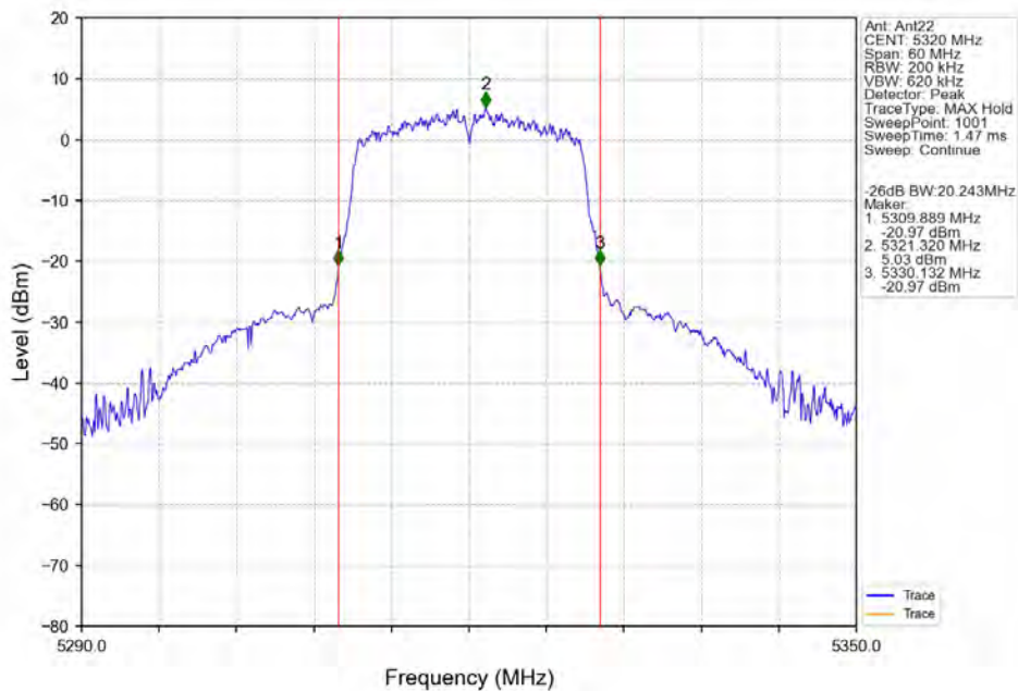
802.11n(HT20)_HCH_5320MHz_Ant22_NTNV
