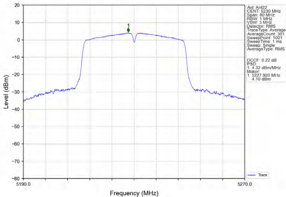
802.11n(HT40)_HCH_5230MHz_Ant22_NTNV
