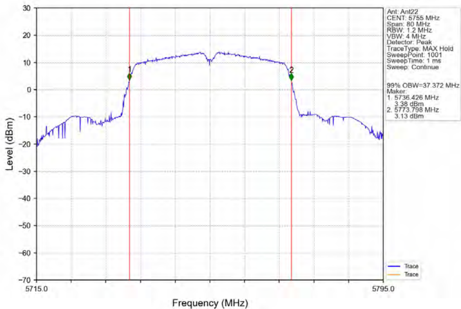
802.11n(HT40)_LCH_5755MHz_Ant22_NTNV
