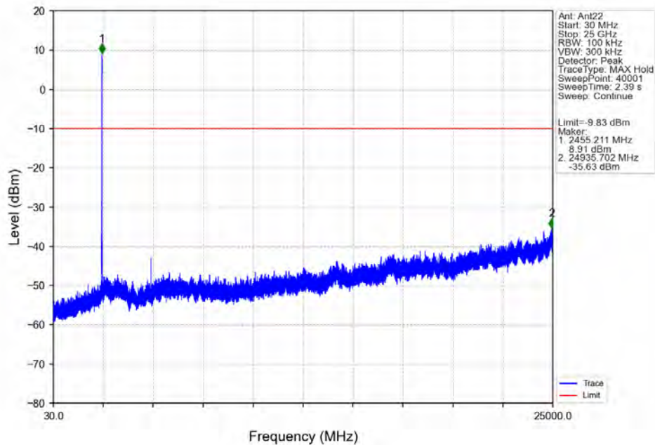
802.11b_HCH_2462MHz_Ant22_NTNV
