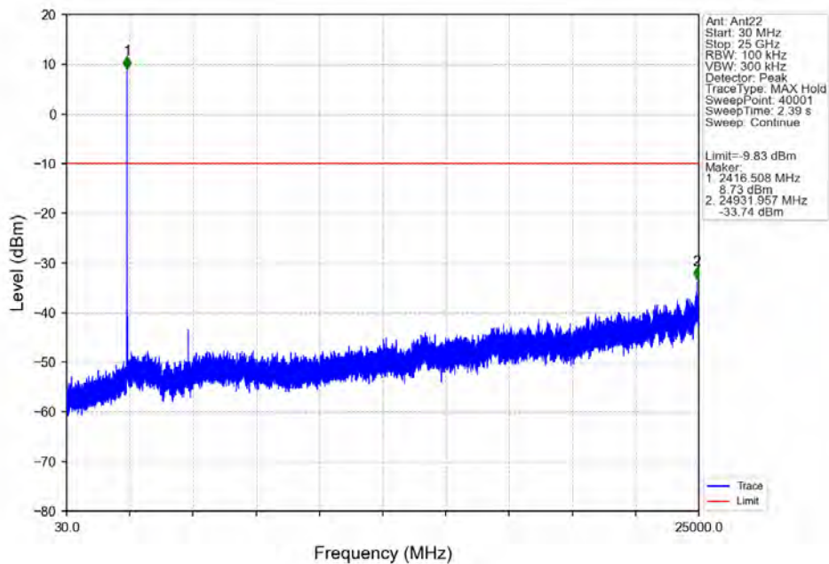
802.11b_LCH_2417MHz_Ant22_NTNV
