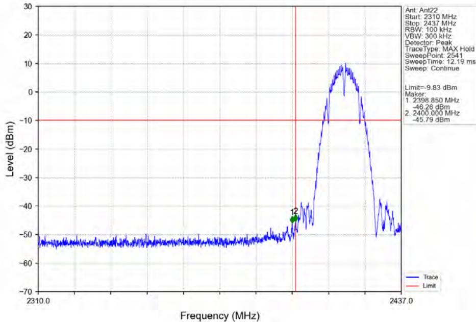
802.11b_LCH_2417MHz_Ant22_NTNV
