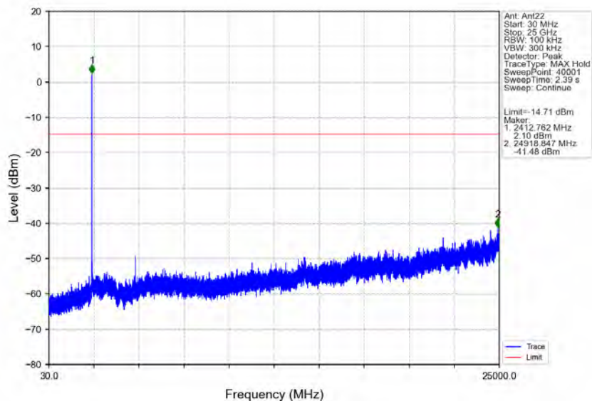
802.11b_LCH_2412MHz_Ant22_NTNV
