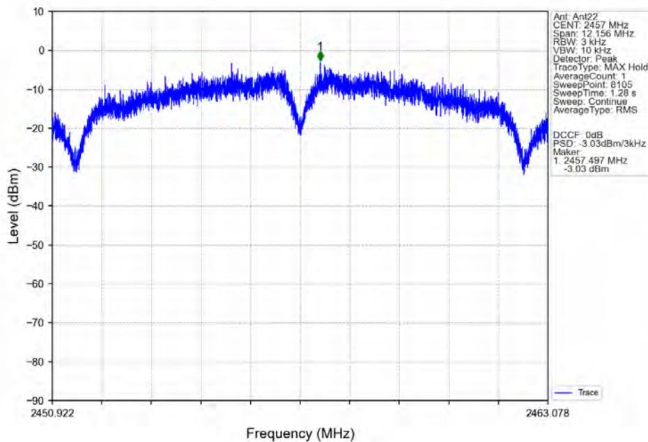
802.11b_HCH_2457MHz_Ant22_NTNV
