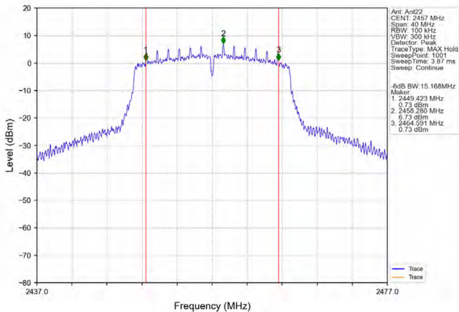
802.11n(HT20)_HCH_2457MHz_Ant22_NTNV
