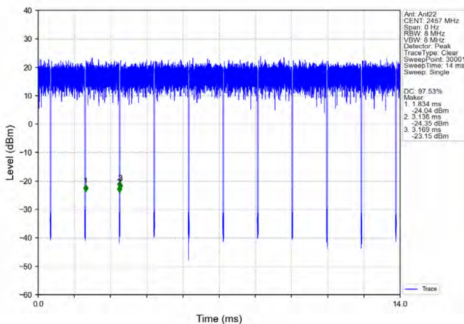
802.11n(HT20)_HCH_2457MHz_Ant22_NTNV
