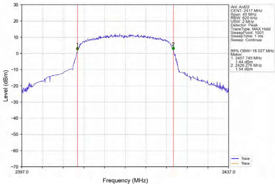
802.11n(HT20)_LCH_2417MHz_Ant22_NTNV
