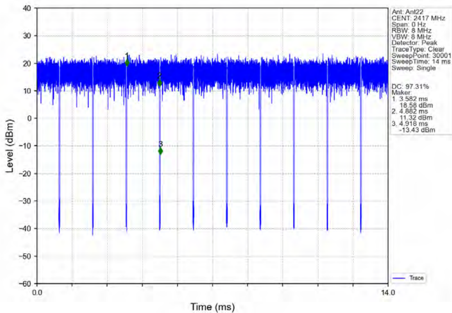
802.11n(HT20)_LCH_2417MHz_Ant22_NTNV
