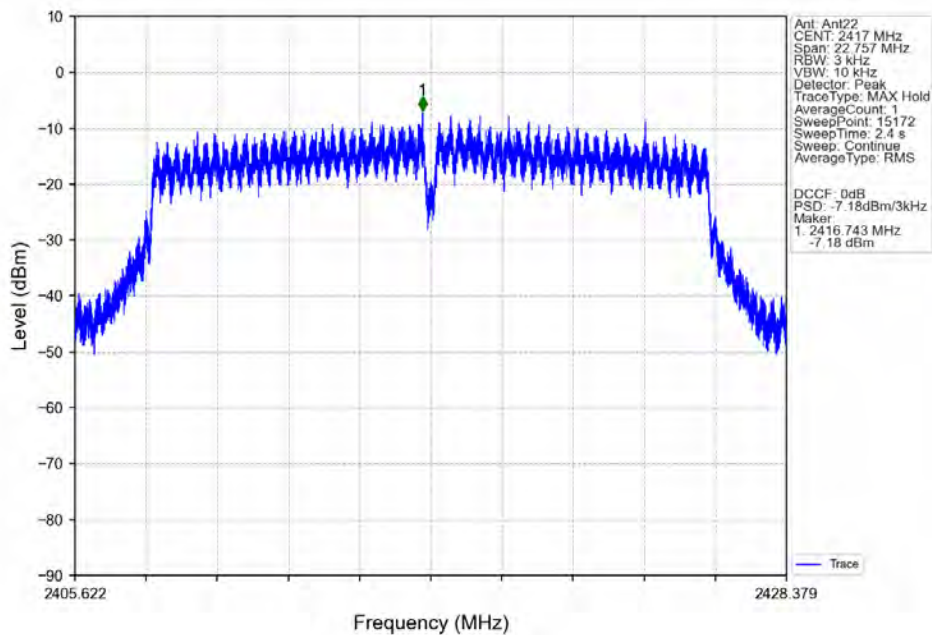
802.11n(HT20)_LCH_2417MHz_Ant22_NTNV
