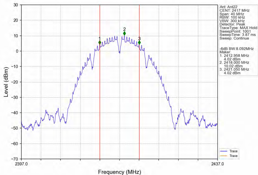
802.11b_LCH_2417MHz_Ant22_NTNV
