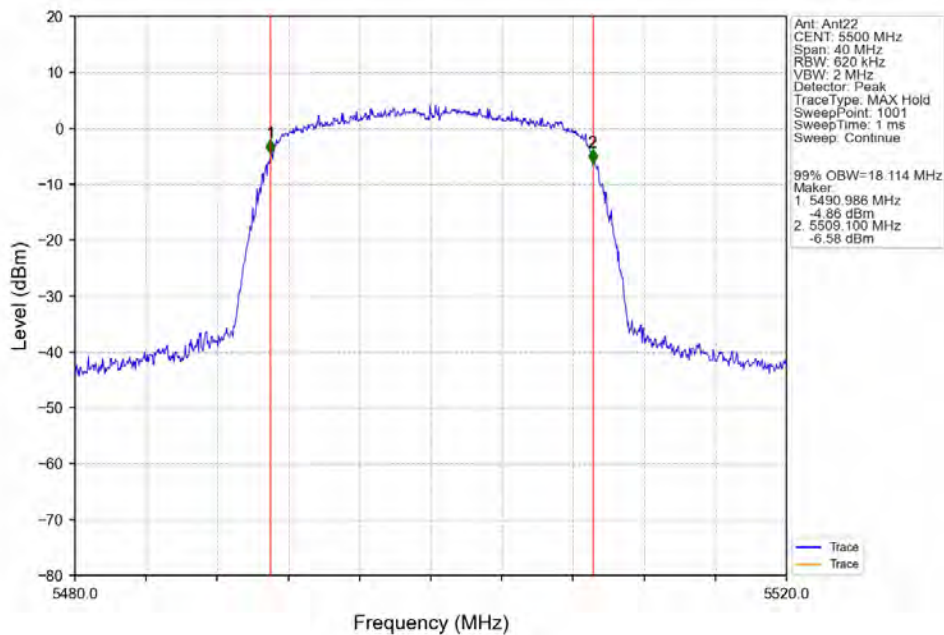
802.11n(HT20)_LCH_5500MHz_Ant22_NTNV
