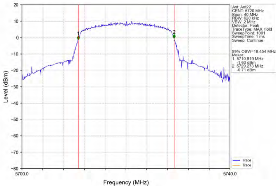
802.11n(HT20)_HCH_5720MHz_Ant22_NTNV
