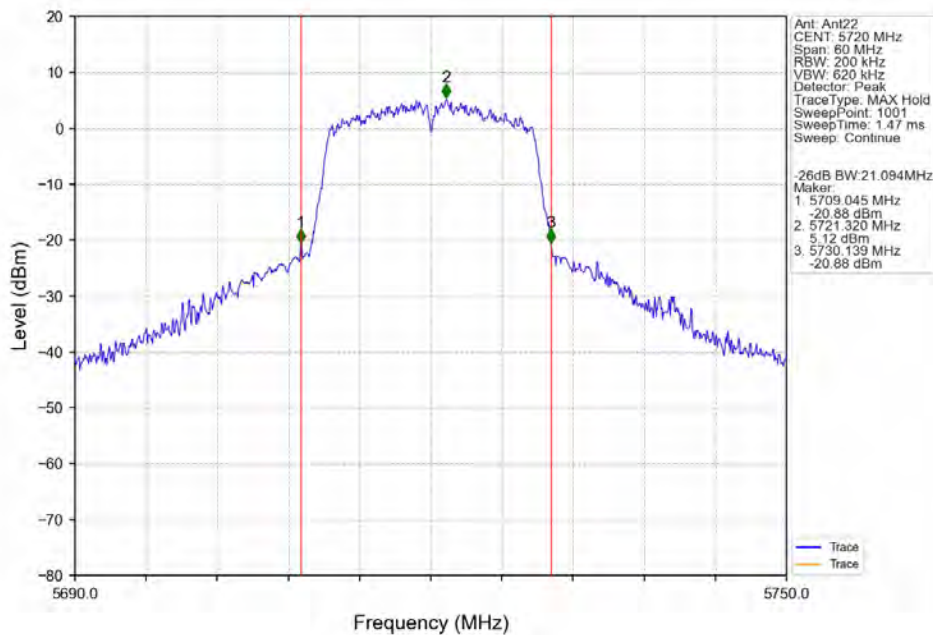
802.11n(HT20)_HCH_5720MHz_Ant22_NTNV
