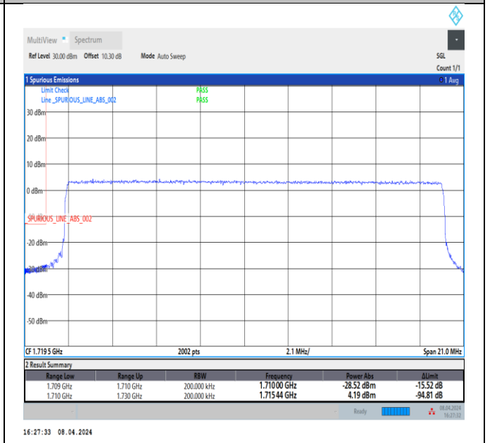
Band66_20MHz_QPSK_132072_100RB#0
