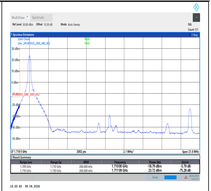
Band66_20MHz_QPSK_132072_1RB#0
