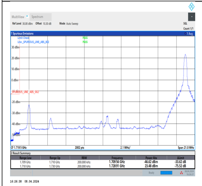
Band66_20MHz_QPSK_132072_1RB#99
