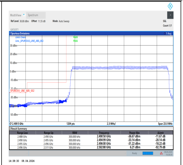
Band41_15MHz_QPSK_39725_75RB#0
