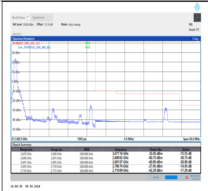
Band41_20MHz_QPSK_41490_1RB#0
