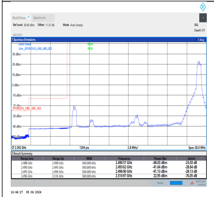
Band41_20MHz_QPSK_39750_1RB#99
