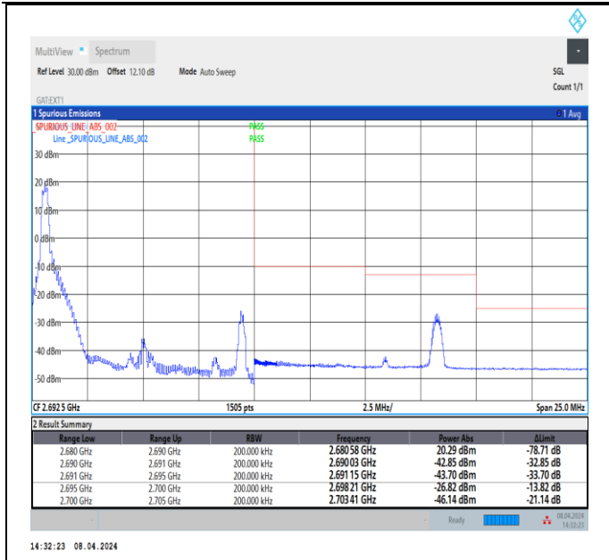
Band41_10MHz_QPSK_41540_1RB#0
