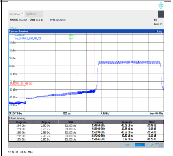
Band38_20MHz_QPSK_37850_100RB#0
