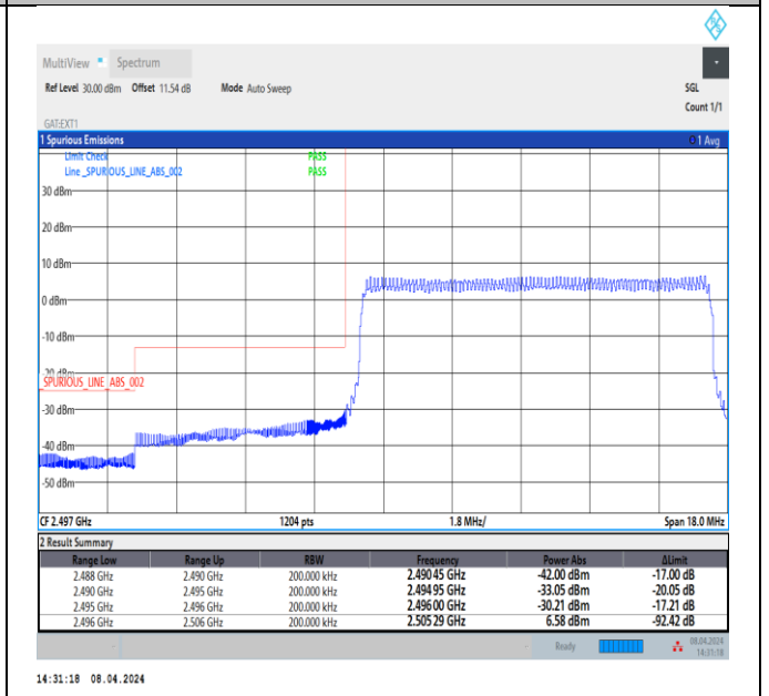
Band41_10MHz_QPSK_39700_50RB#0
