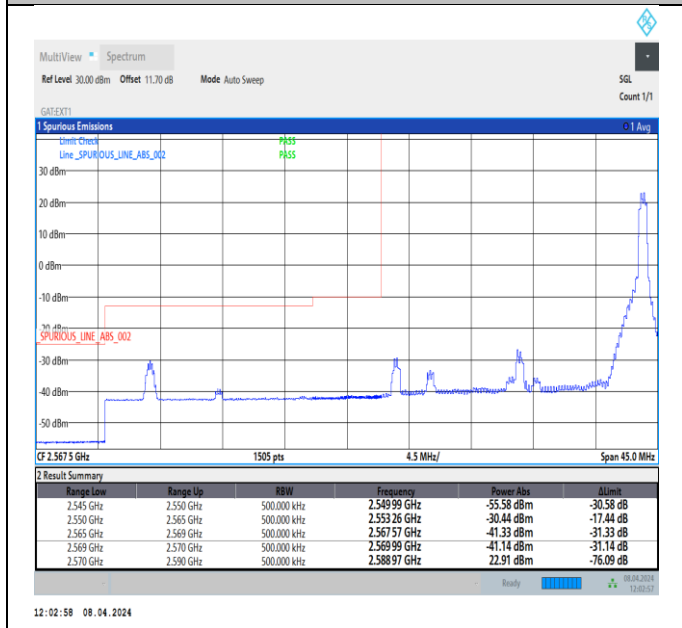
Band38_20MHz_QPSK_37850_1RB#99
