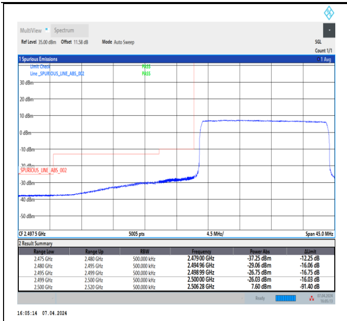
Band7_20MHz_QPSK_20850_100RB#0
