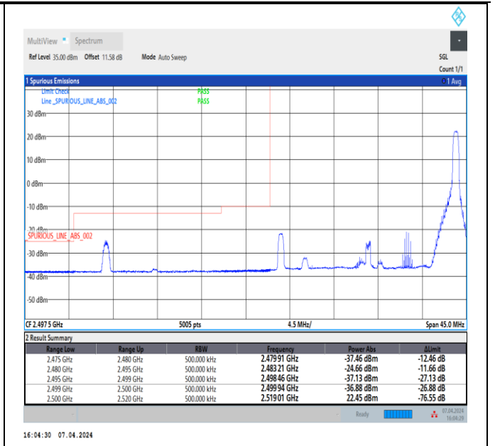
Band7_20MHz_16QAM_20850_1RB#99
