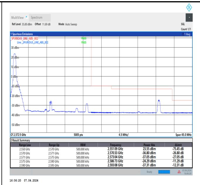
Band7_20MHz_QPSK_21350_1RB#0
