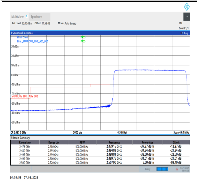
Band7_20MHz_64QAM_20850_100RB#0
