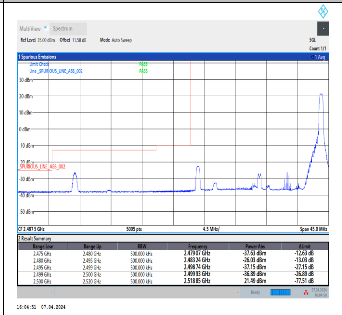
Band7_20MHz_64QAM_20850_1RB#99
