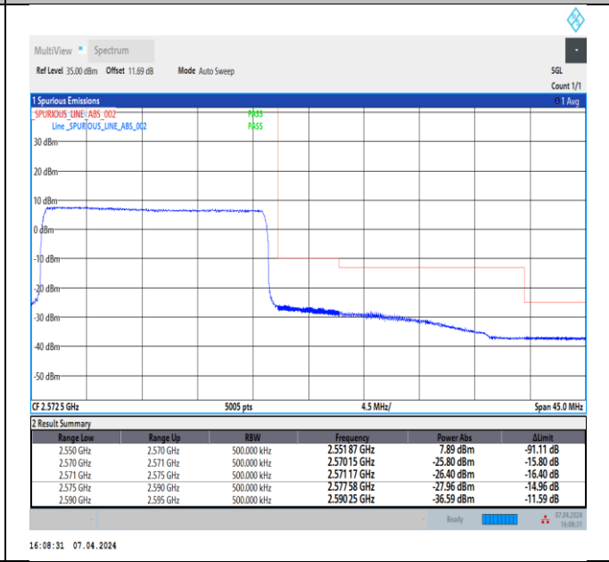
Band7_20MHz_QPSK_21350_100RB#0
