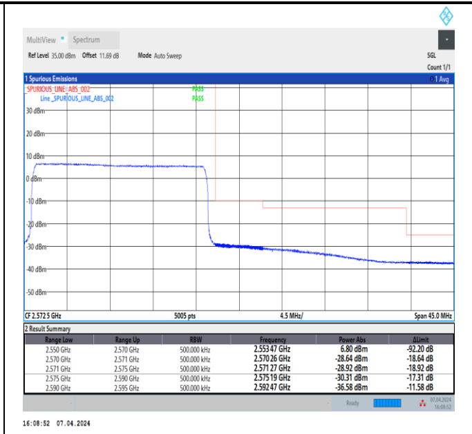
Band7_20MHz_16QAM_21350_100RB#0
