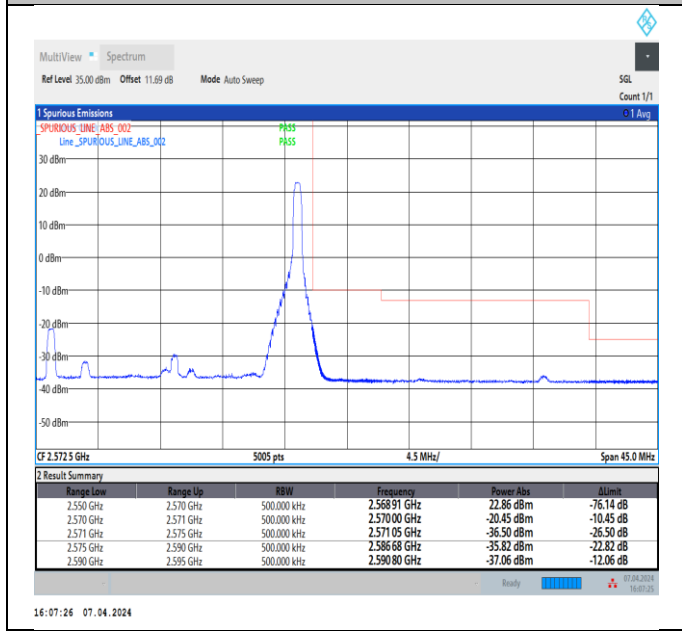
Band7_20MHz_QPSK_21350_1RB#99
