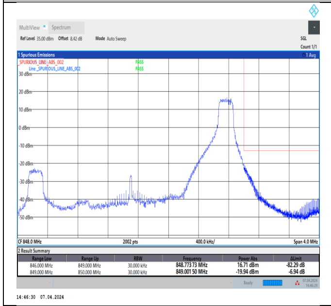
Band5_3MHz_64QAM_20635_1RB#14
