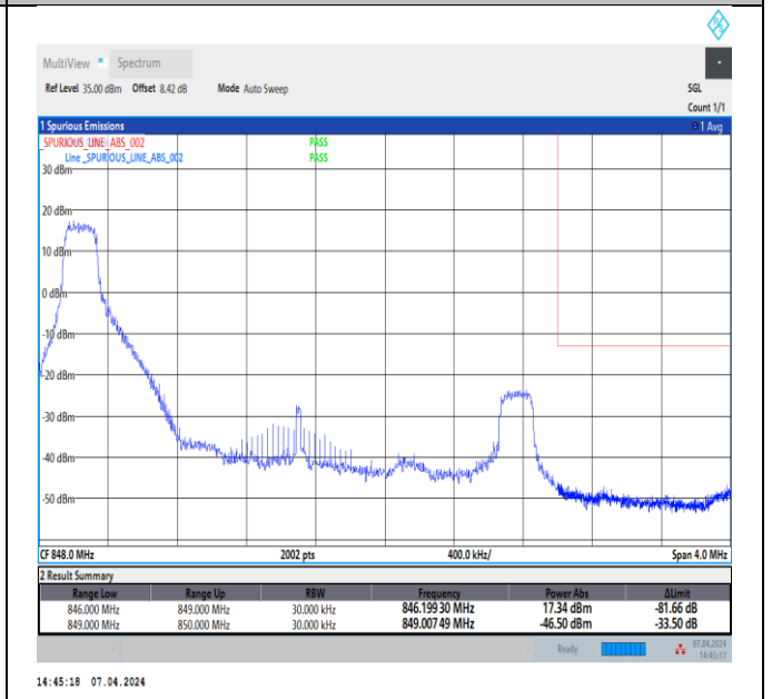
Band5_3MHz_16QAM_20635_1RB#0
