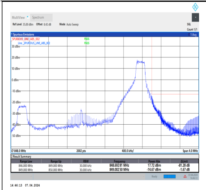
Band5_3MHz_16QAM_20635_1RB#14
