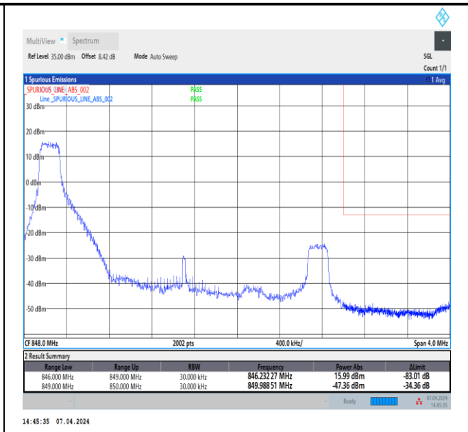
Band5_3MHz_64QAM_20635_1RB#0
