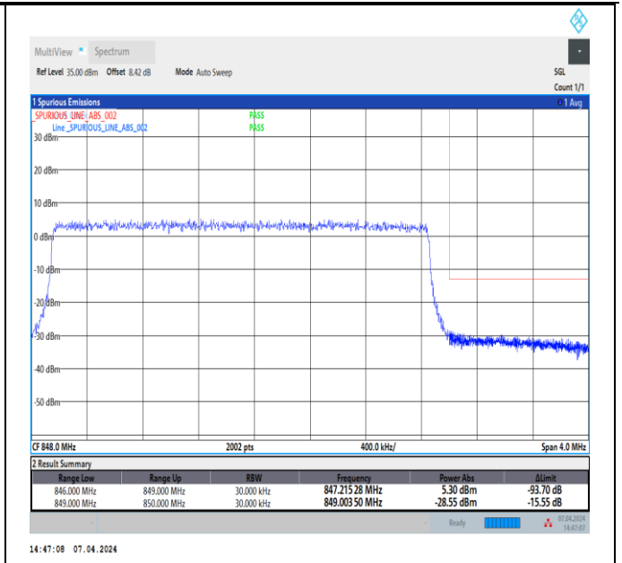
Band5_3MHz_16QAM_20635_15RB#0
