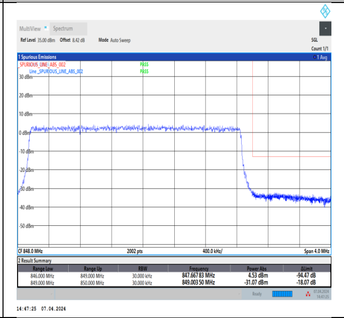
Band5_3MHz_64QAM_20635_15RB#0
