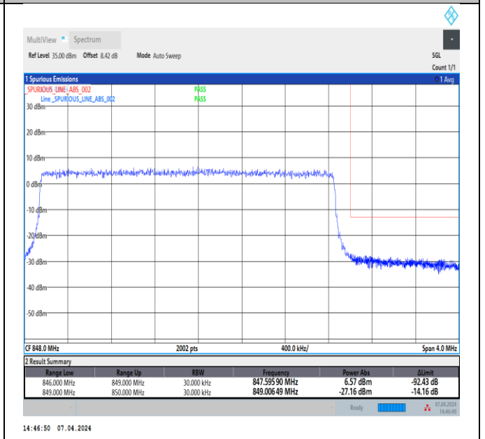
Band5_3MHz_QPSK_20635_15RB#0
