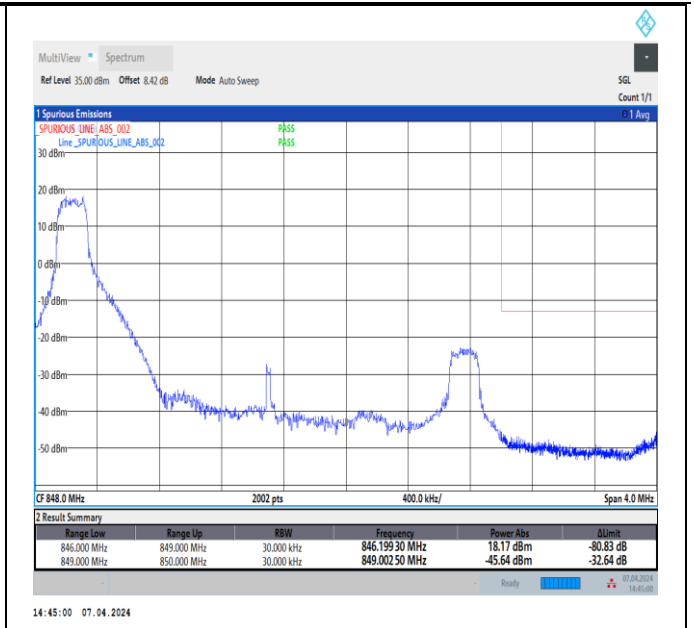
Band5_3MHz_QPSK_20635_1RB#0
