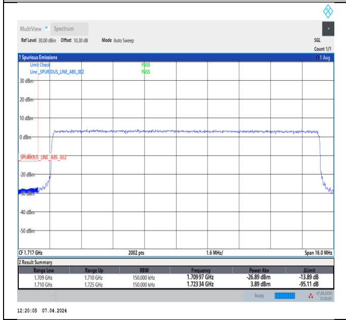
Band4_15MHz_QPSK_2025_75RB#0
