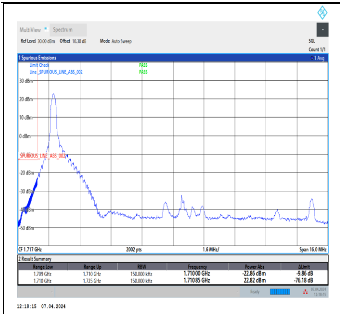
Band4_15MHz_QPSK_2025_1RB#0
