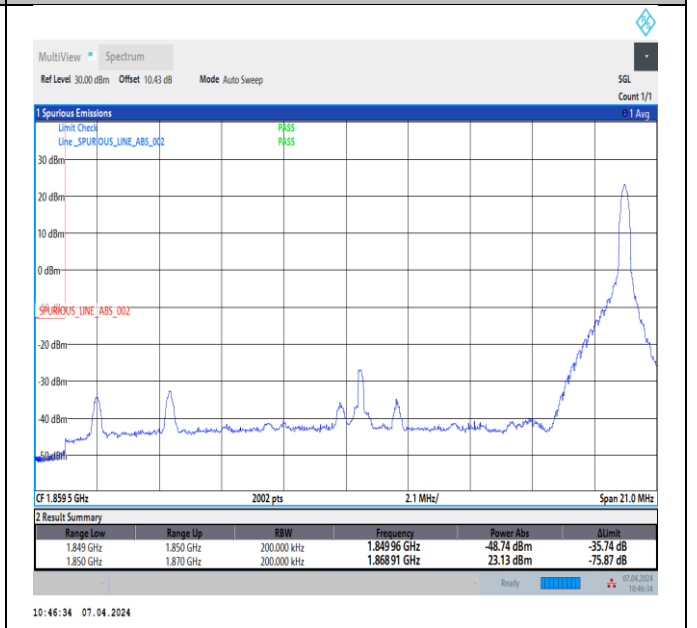
Band2_20MHz_QPSK_18700_1RB#99
