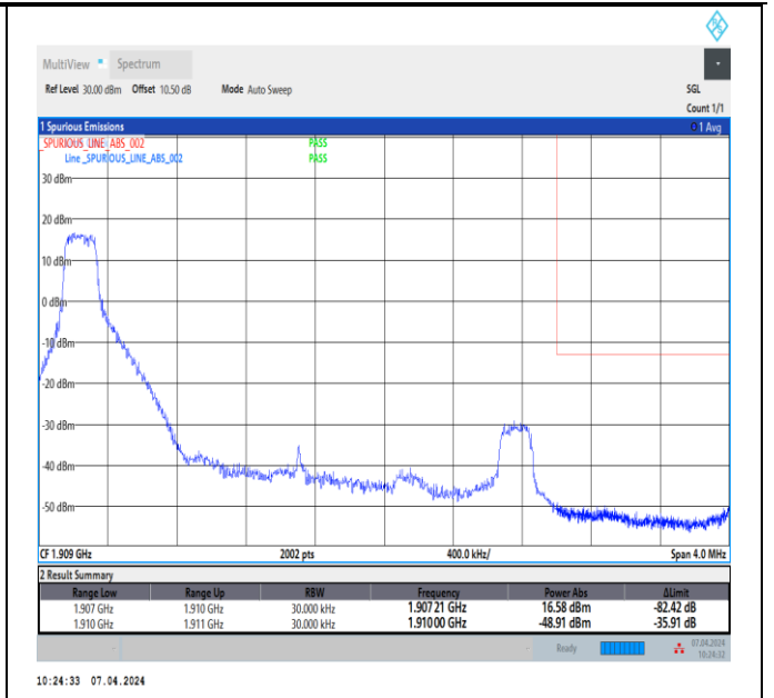
Band2_3MHz_QPSK_19185_1RB#0
