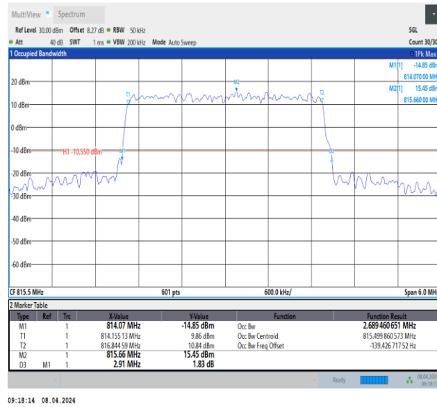
26(814-824)-3MHz-QPSK-26705-15RB#0-PASS
