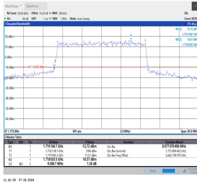
Band4-10MHz-QPSK-20000-50RB#0-PASS
