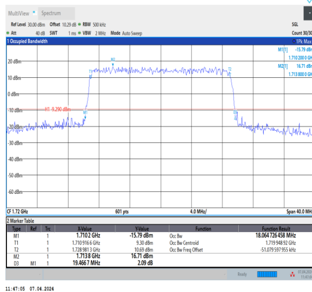
Band4-20MHz-QPSK-20050-100RB#0-PASS
