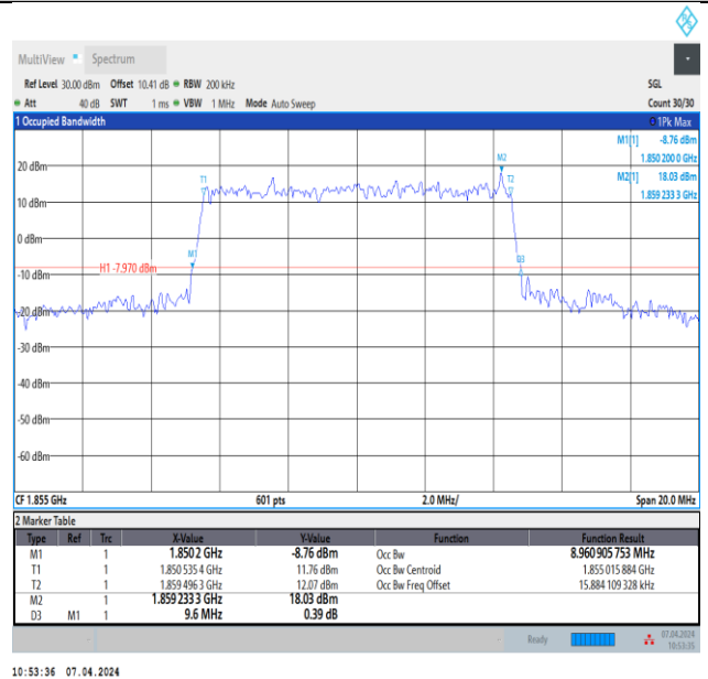
Band2-10MHz-QPSK-18650-50RB#0-PASS
