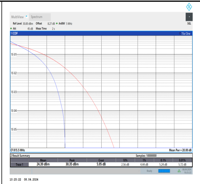
26(814-824)-3MHz-QPSK-26705-15RB#0-PASS
