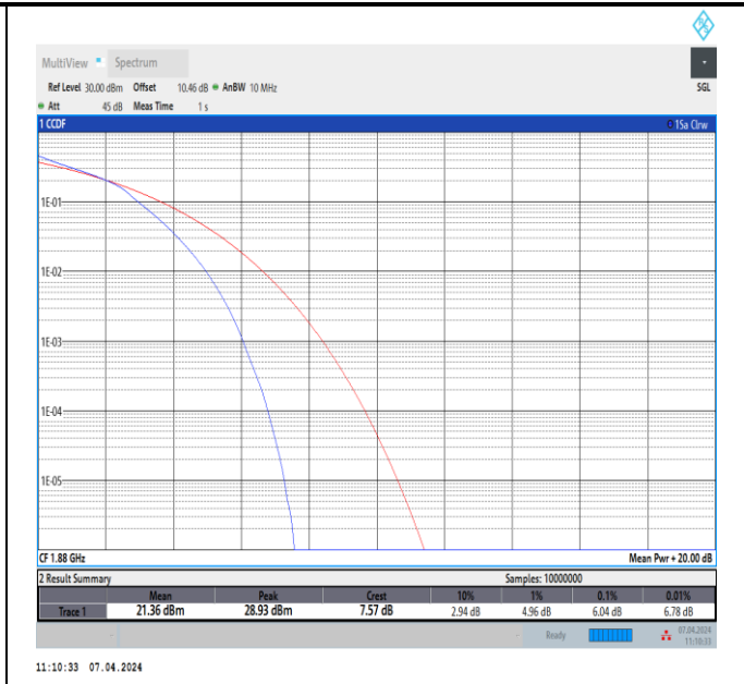
Band2-10MHz-16QAM-18900-50RB#0-PASS
