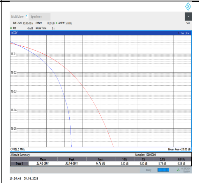
26(814-824)-3MHz-QPSK-26775-15RB#0-PASS
