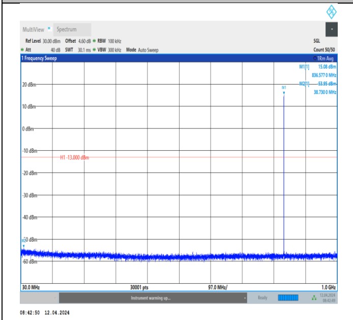
GSM850-190-5-30~1000MHz-PASS
