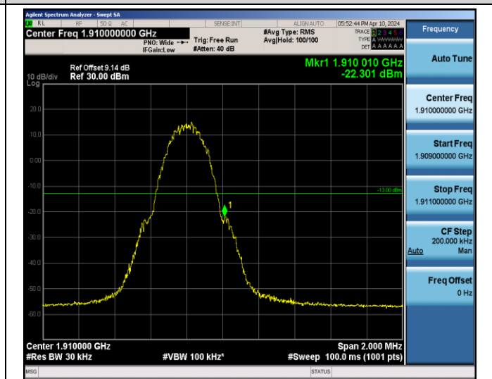
GPRS1900-810-0
