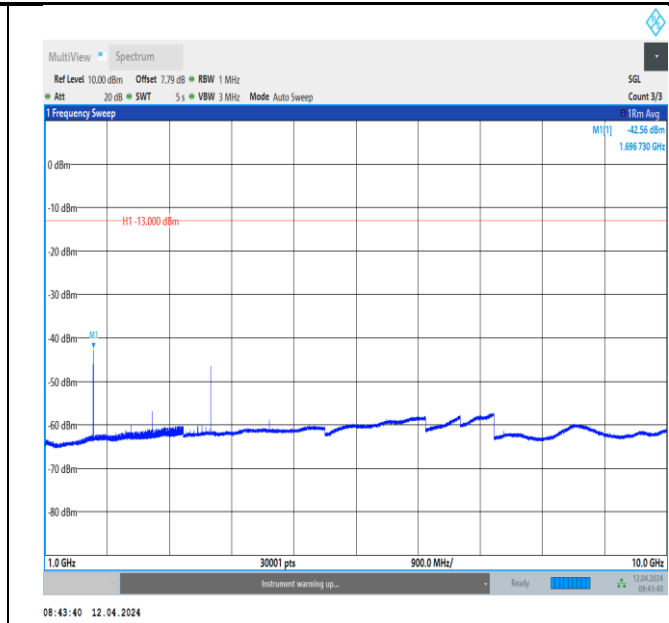
GSM850-251-5-1000~10000MHz-PASS
