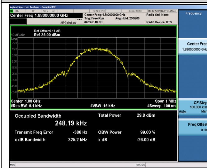
EGPRS1900-661-2-0.3252
