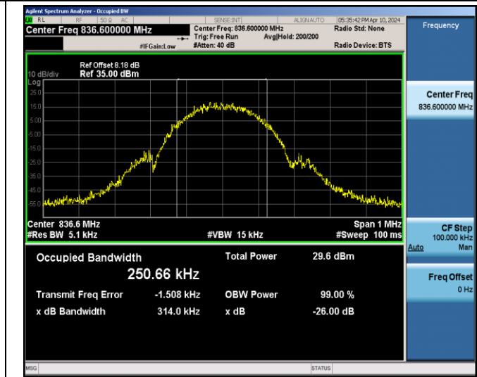
EGPRS850-190-8-0.3140
