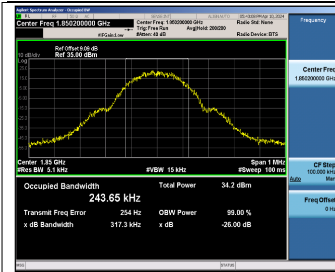
GPRS1900-512-0-0.3173
