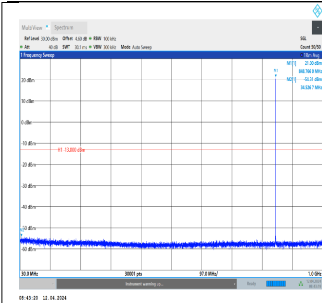
GSM850-251-5-30~1000MHz-PASS
