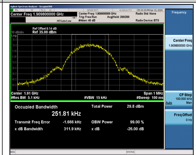
EGPRS1900-810-2-0.3119
