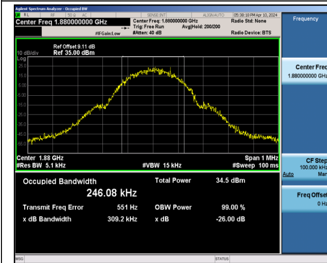
GSM1900-661-0-0.3092
