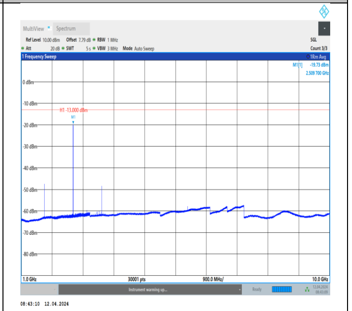
GSM850-190-5-1000~10000MHz-PASS
