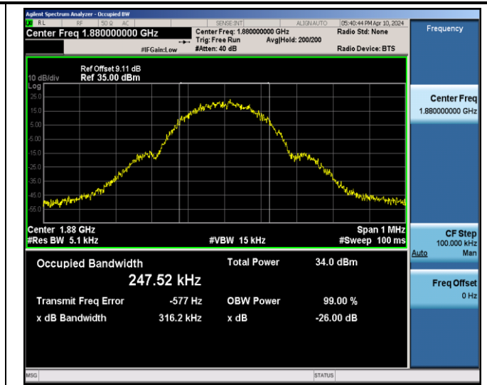
GPRS1900-661-0-0.3162
