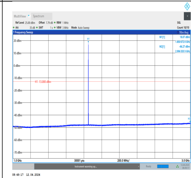
GSM1900-512-0-1000~3000MHz-PASS
