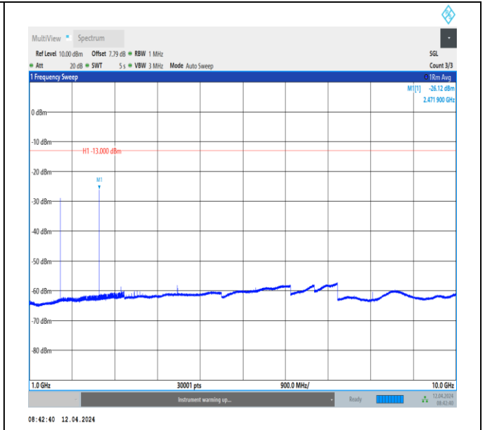
GSM850-128-5-1000~10000MHz-PASS
