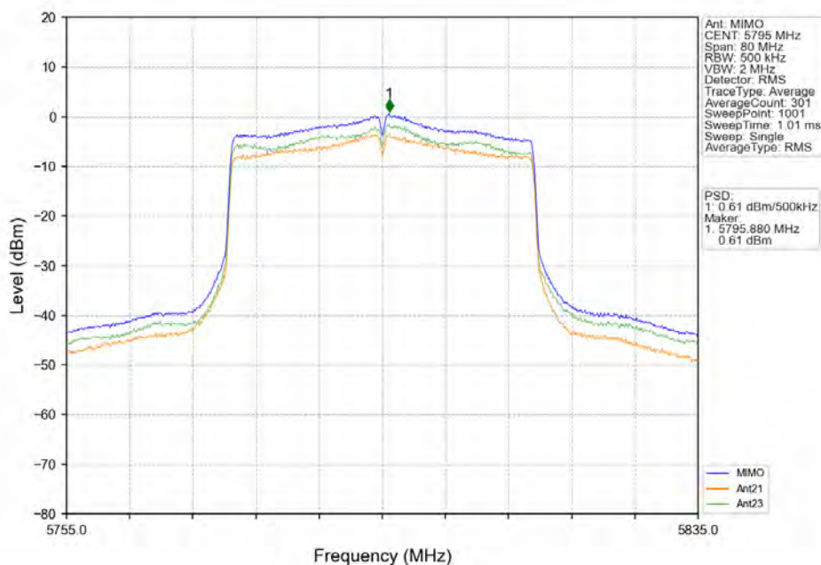
802.11ax(HE40) HCH 5795MHz RU484 Left MIMO NTV
