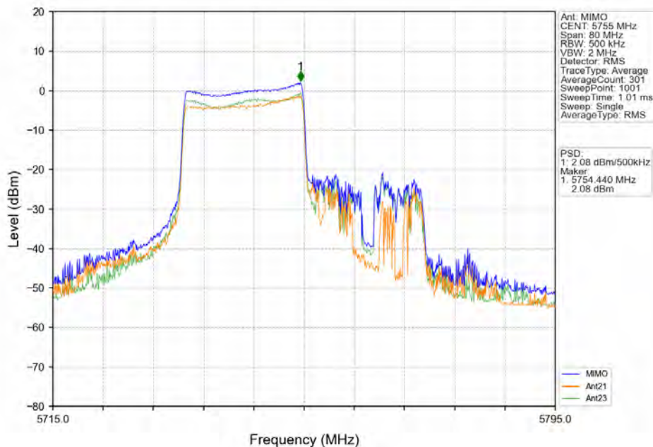
802.11ax(HE40) LCH_5755MHz_RU242_Left_MIMO_NTNV
