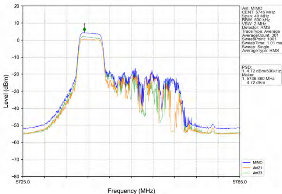
802.11ax(HE20) LCH 5745MHz RU52 Left MIMO NTNV
