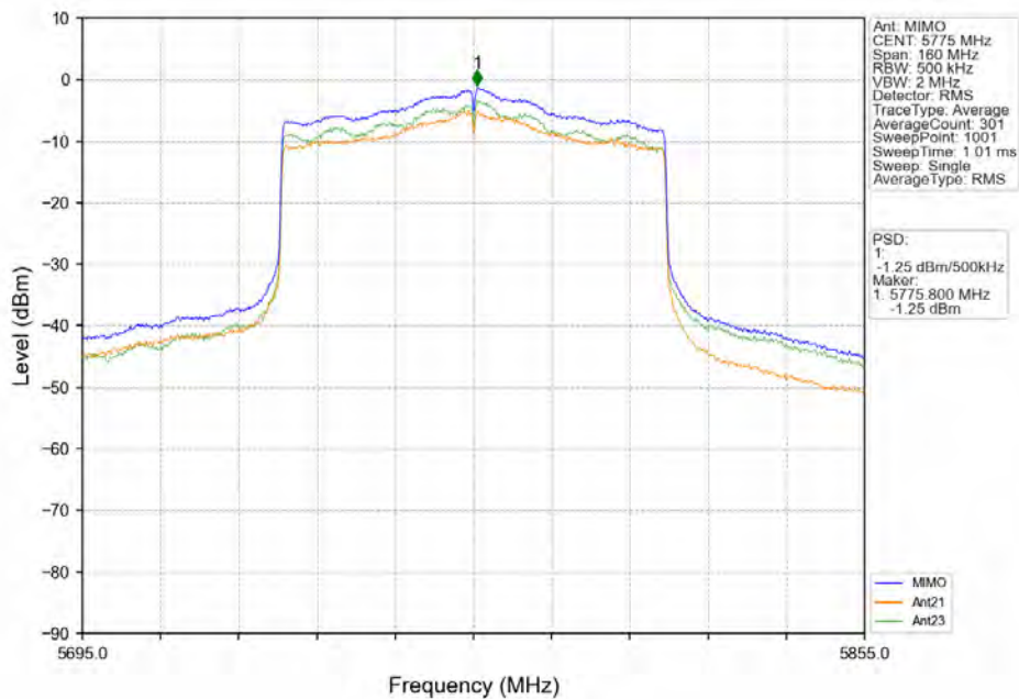
802.11ax(HE80) MCH 5775MHz RU996 Left MIMO NTNV
