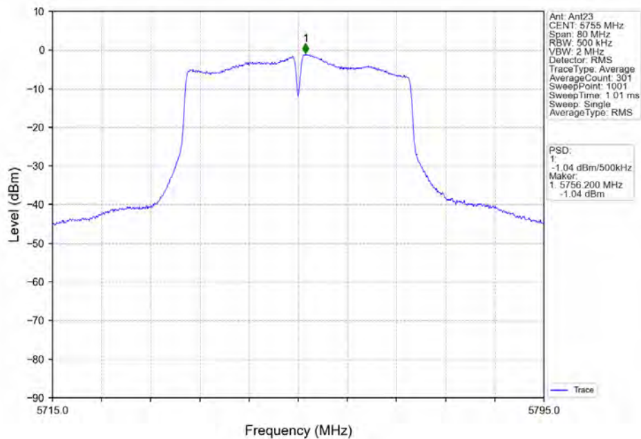
802.11n(HT40) LCH_5755MHz_Ant23_NTNV
