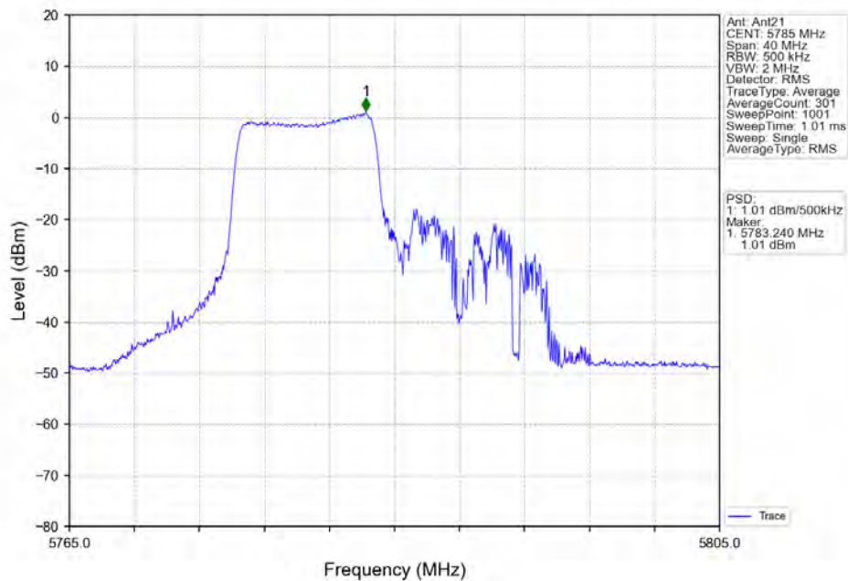
802.11ax(HE20) MCH 5785MHz RU106 Left Ant21_NTNV
