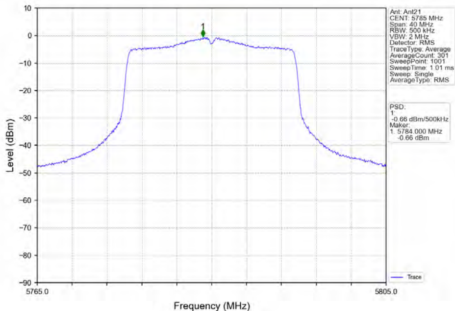
802.11ax(HE20) MCH 5785MHz RU242 Left Ant21 NTNV
