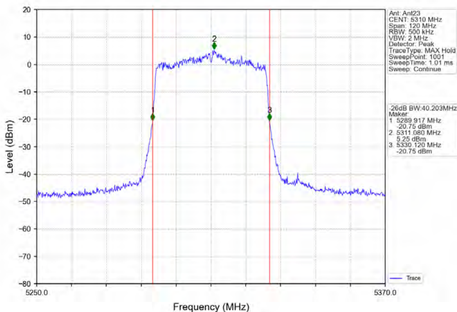
802.11ax(HE40) HCH 5310MHz RU484 Left Ant23 NTN
