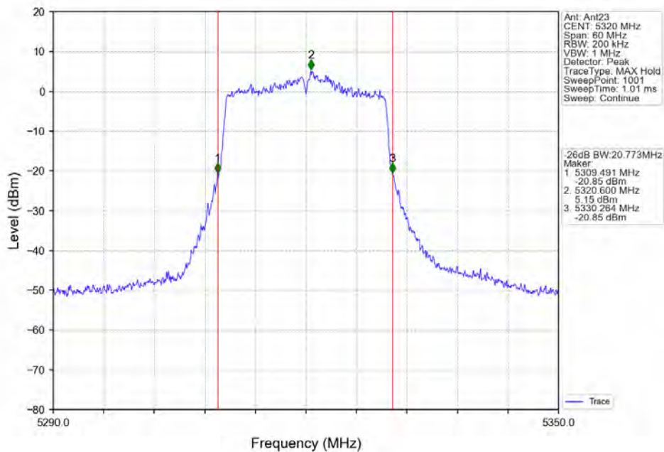
802.11ax(HE20) HCH 5320MHz RU242 Left Ant23 NTNV
