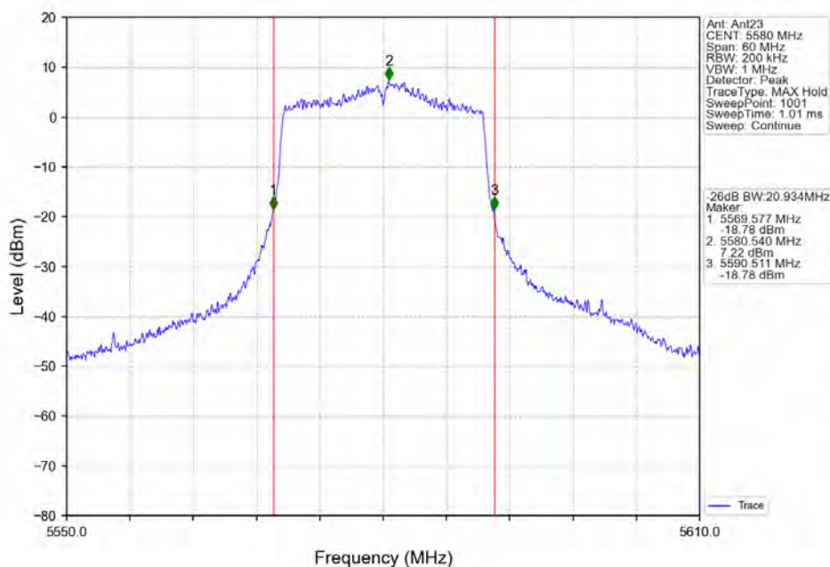
802.11ax(HE20) MCH 5580MHz RU242 Left Ant23 NTVN
