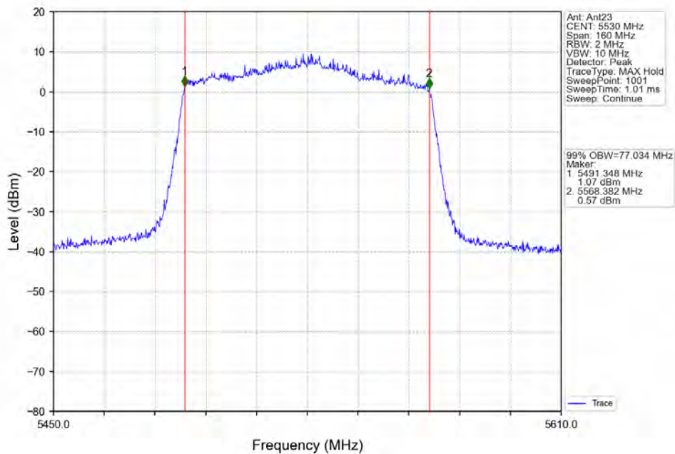
802.11ax(HE80) LCH_5530MHz_RU996_Left_Ant23_NTNV
