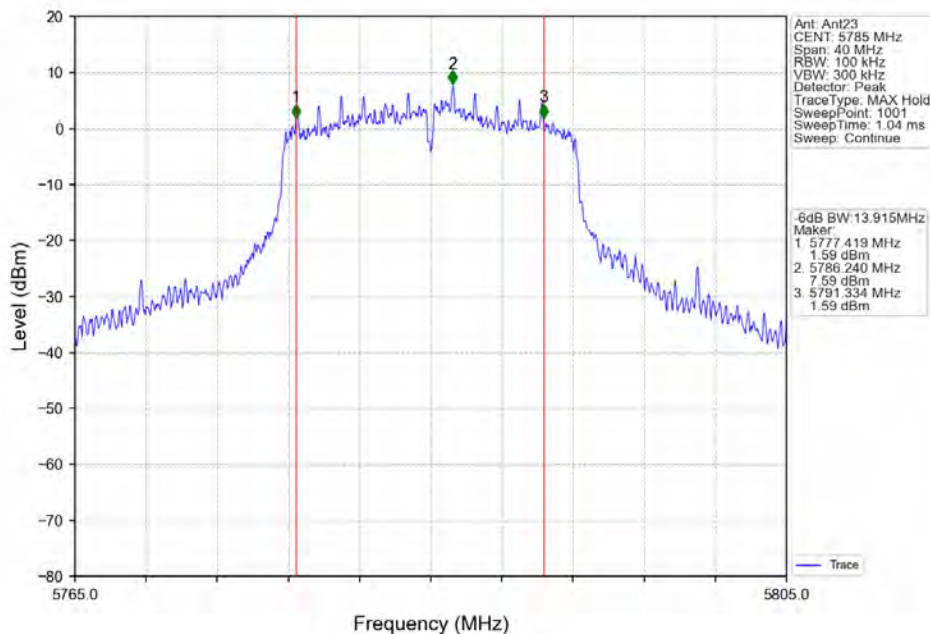
802.11a MCH_5785MHz_Ant23_NTNV
