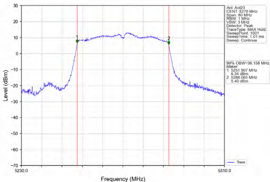
802.11n(HT40) LCH_5270MHz_Ant23_NTNV
