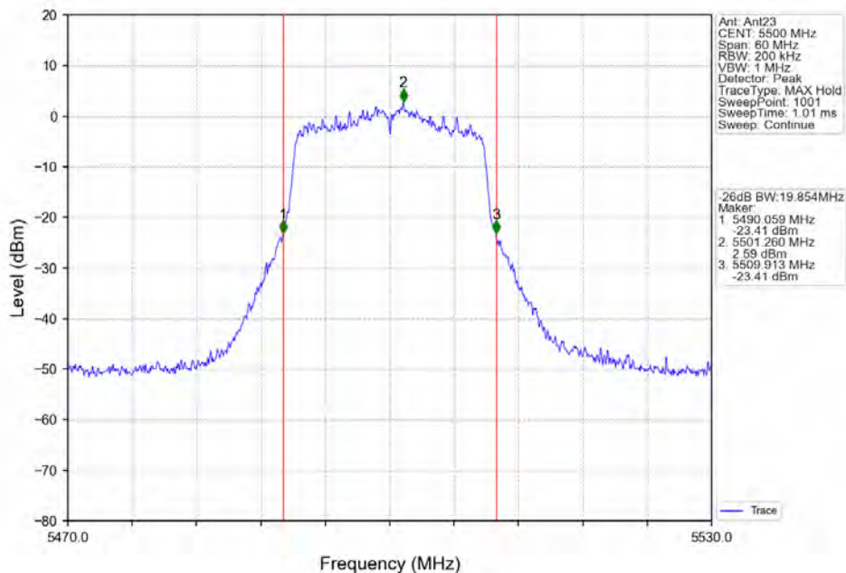
802.11n(HT20) LCH_5500MHz_Ant23_NTNV
