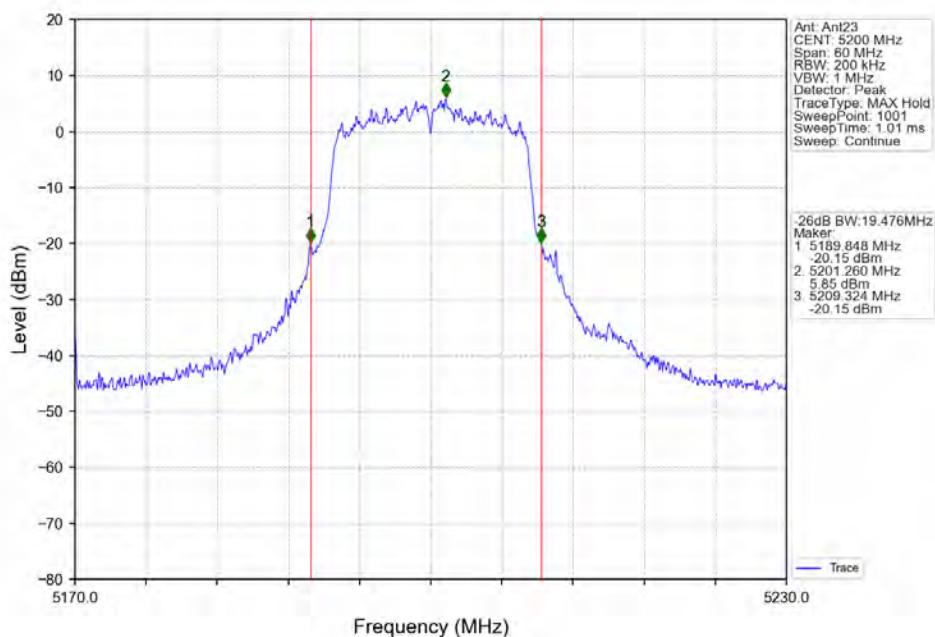
802.11a MCH_5200MHz_Ant23_NTNV
