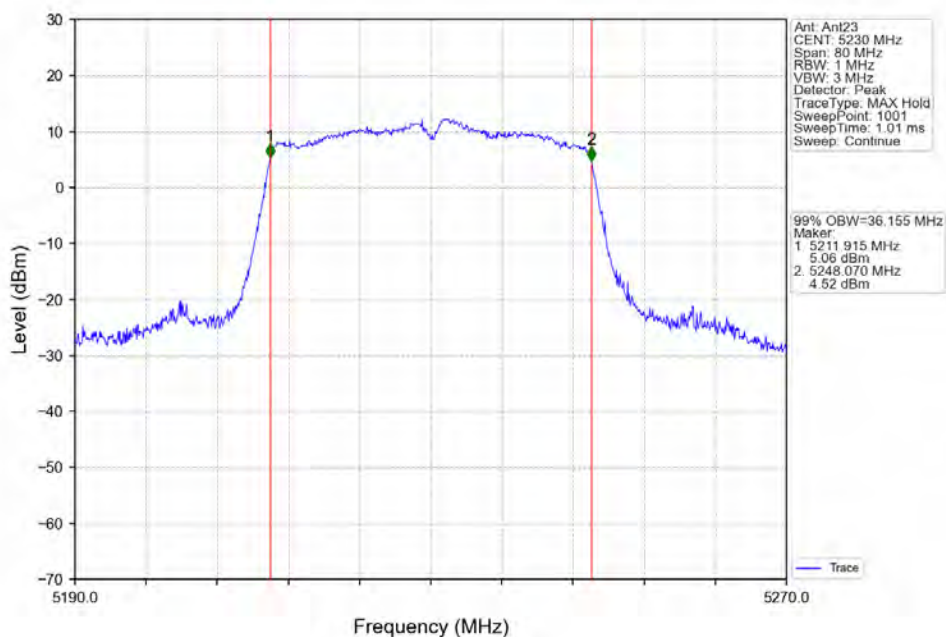
802.11ac(VHT40) HCH_5230MHz_Ant23_NTNV
