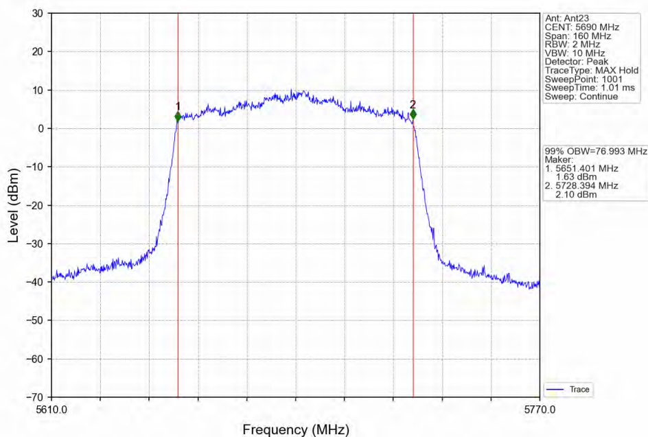
802.11ax(HE80) HCH 5690MHz RU996 Left Ant23 NTNV
