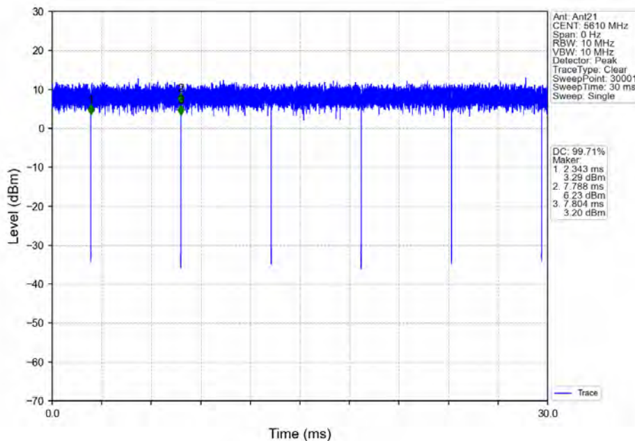
802.11ax(HE80)_HCH_5610MHz_RU996_Left_Ant21_NTNV
