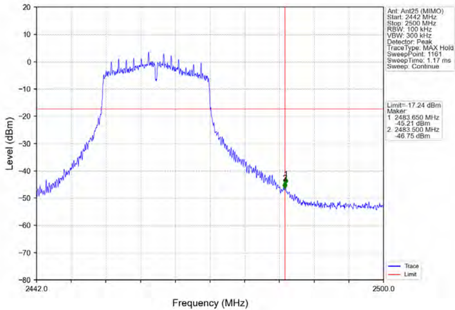
802.11ac(VHT20) HCH 2462MHz Ant25 (MIMO) NTN
