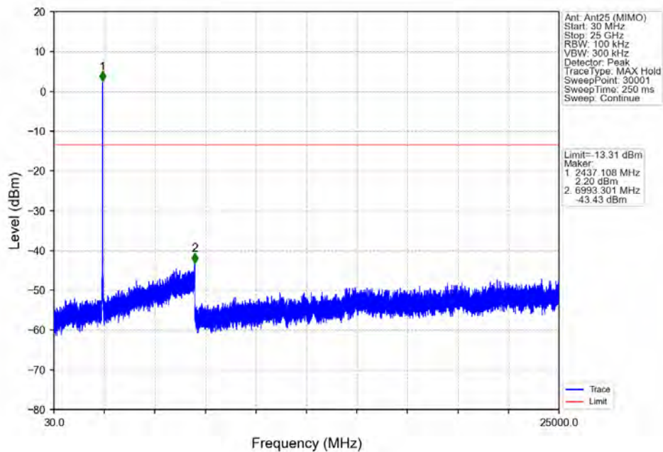
802.11n(HT20)_MCH_2437MHz_Ant25 (MIMO)_NTNV
