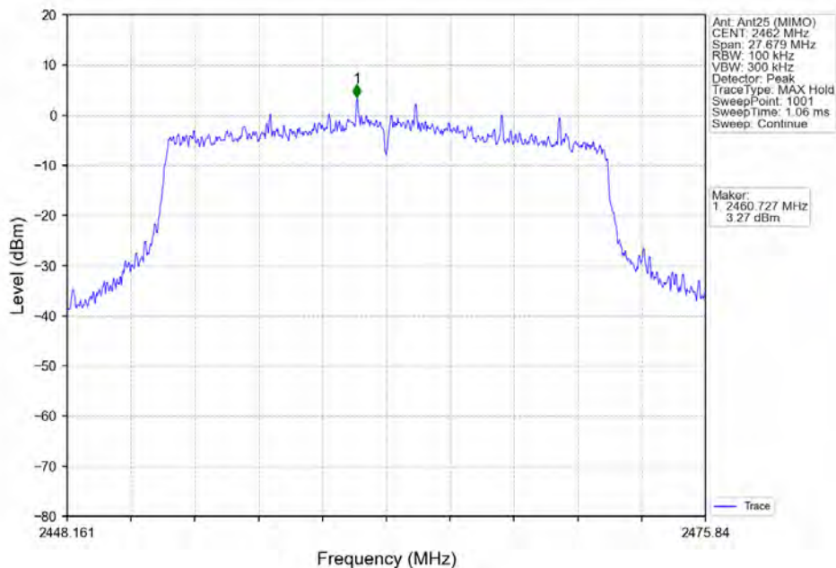
802.11ax(HEW20) HCH 2462MHz RU242 Left Ant25 (MIMO) NTV
