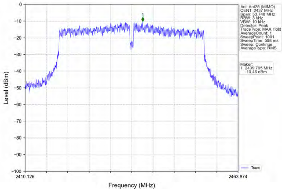
802.11n(HT40)_MCH_2437MHz_Ant25 (MIMO)_NTNV
