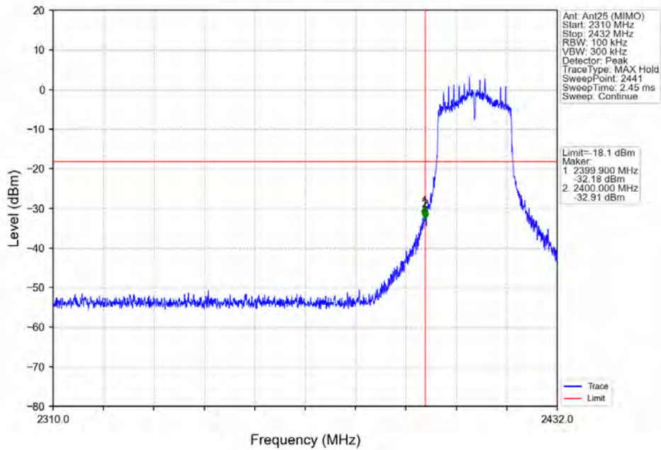
802.11n(HT20) LCH 2412MHz Ant25 (MIMO) NTVN
