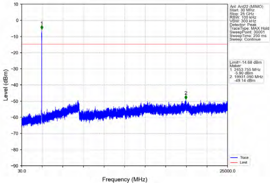
802.11n(HT40)_HCH_2452MHz_Ant22 (MIMO)_NTNV
