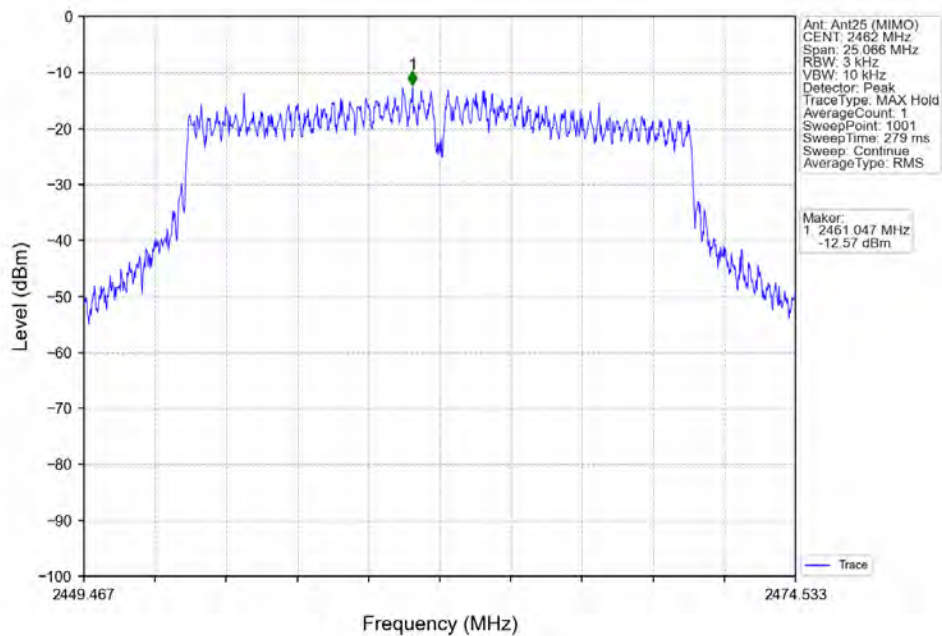
802.11n(HT20)_HCH_2462MHz_Ant25 (MIMO)_NTNV
