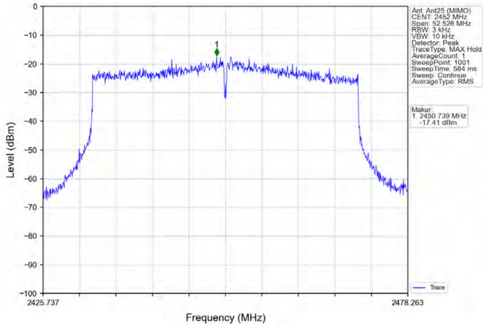
802.11ax(HEW40) HCH 2452MHz RU484 Left MIMO NTVN
