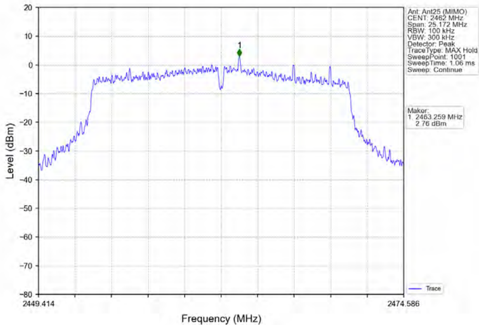
802.11ac(VHT20) HCH 2462MHz Ant25 (MIMO) NTNV
