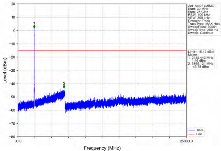
802.11n(HT40)_MCH_2437MHz_Ant25 (MIMO)_NTNV
