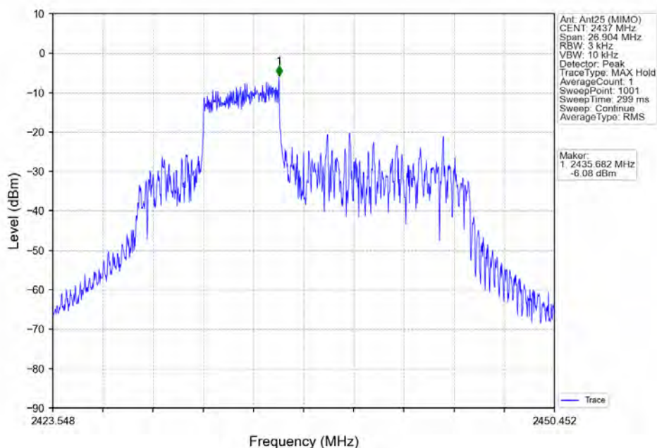
802.11ax(HEW20) MCH 2437MHz RU52 Mid MIMO NTNV
