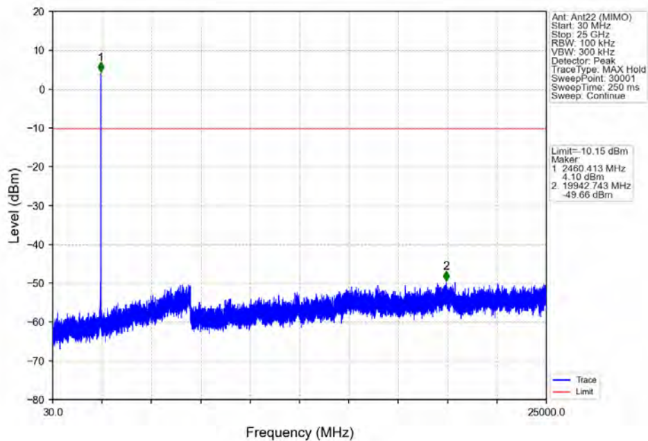
802.11b_HCH_2462MHz_Ant22 (MIMO) NTNV
