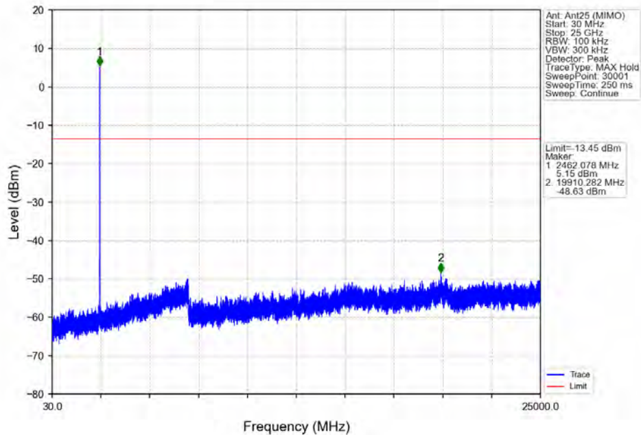
802.11b_HCH_2462MHz_Ant25 (MIMO)_NTNV
