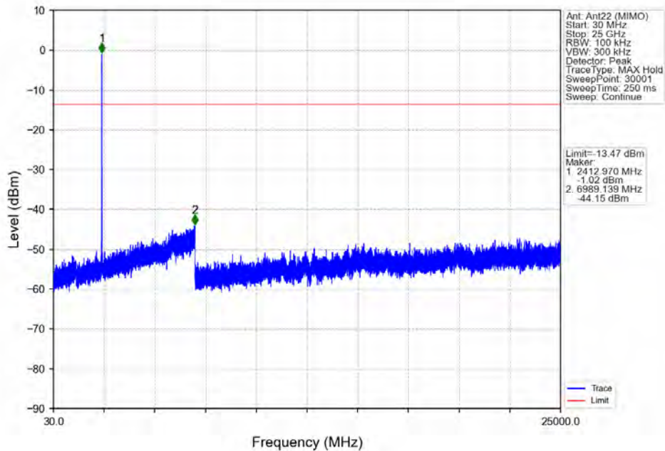
802.11n(HT20) LCH 2412MHz Ant22 (MIMO) NTNV
