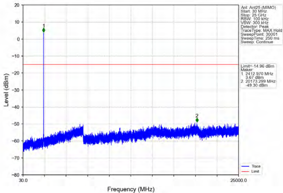
802.11b_LCH_2412MHz_Ant25 (MIMO) NTN
