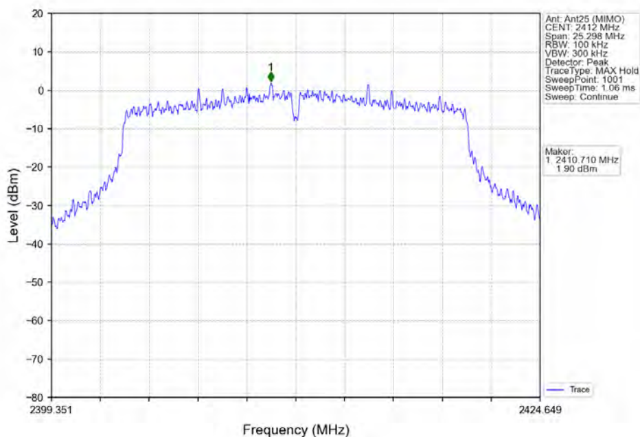
802.11n(HT20) LCH 2412MHz Ant25 (MIMO) NTNV
