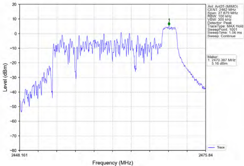
802.11ax(HEW20) HCH 2462MHz RU26_Right_Ant25 (MIMO) NTVN
