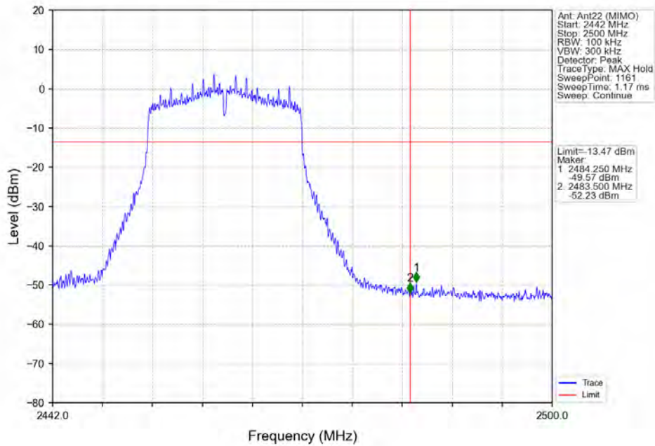
802.11n(HT20)_HCH_2462MHz_Ant22 (MIMO)_NTNV
