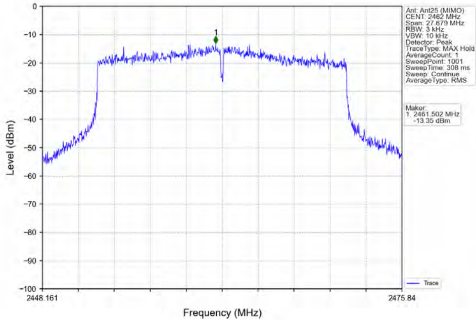
802.11ax(HEW20) HCH 2462MHz RU242 Left MIMO NTN
