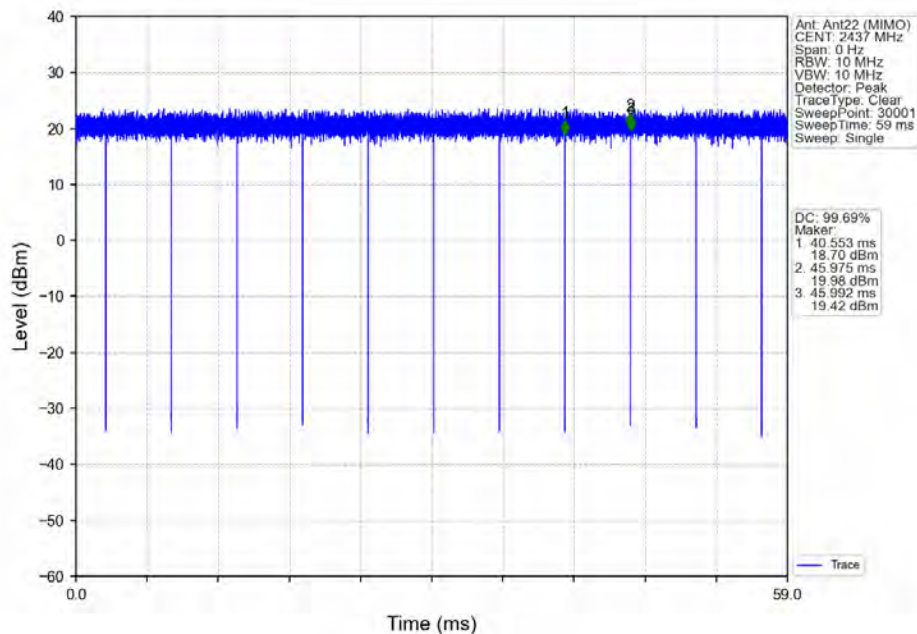
802.11n(HT20)_MCH_2437MHz_Ant22 (MIMO)_NTNV
