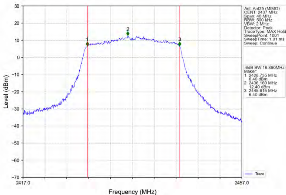
802.11ac(VHT20) MCH 2437MHz Ant25 (MIMO) NTNV
