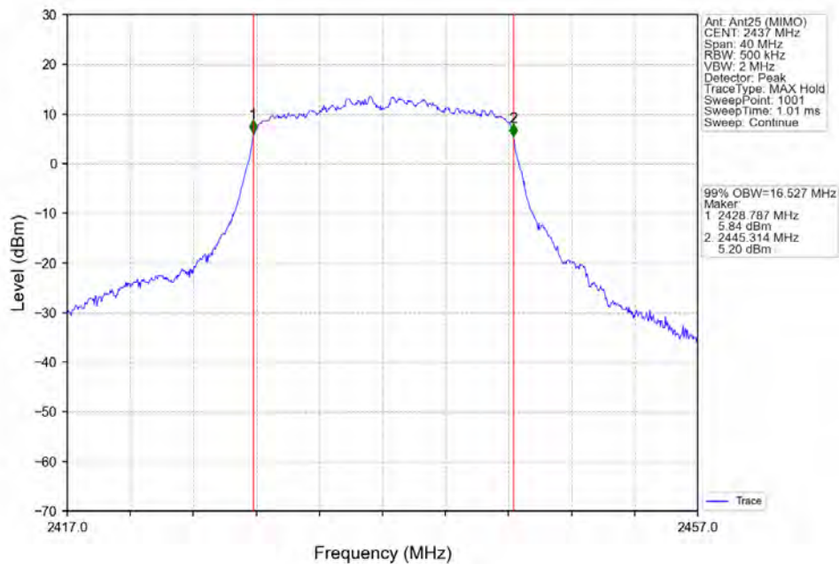
802.11g_MCH_2437MHz_Ant25 (MIMO)_NTNV
