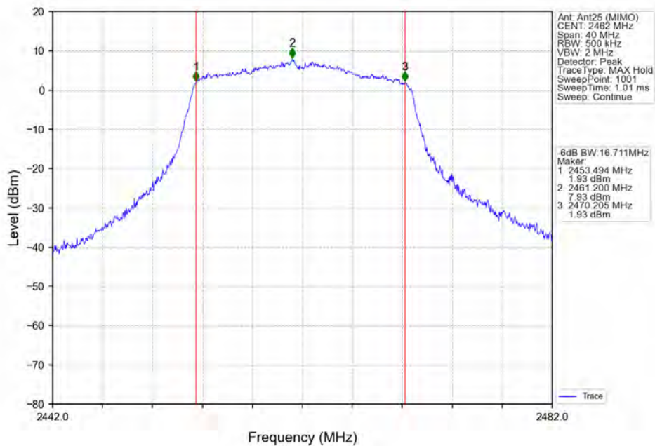
802.11n(HT20)_HCH_2462MHz_Ant25 (MIMO)_NTNV
