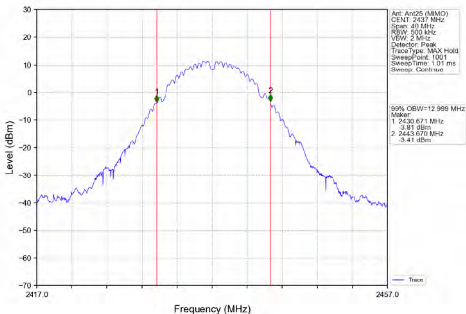
802.11b_MCH_2437MHz_Ant25 (MIMO)_NTNV
