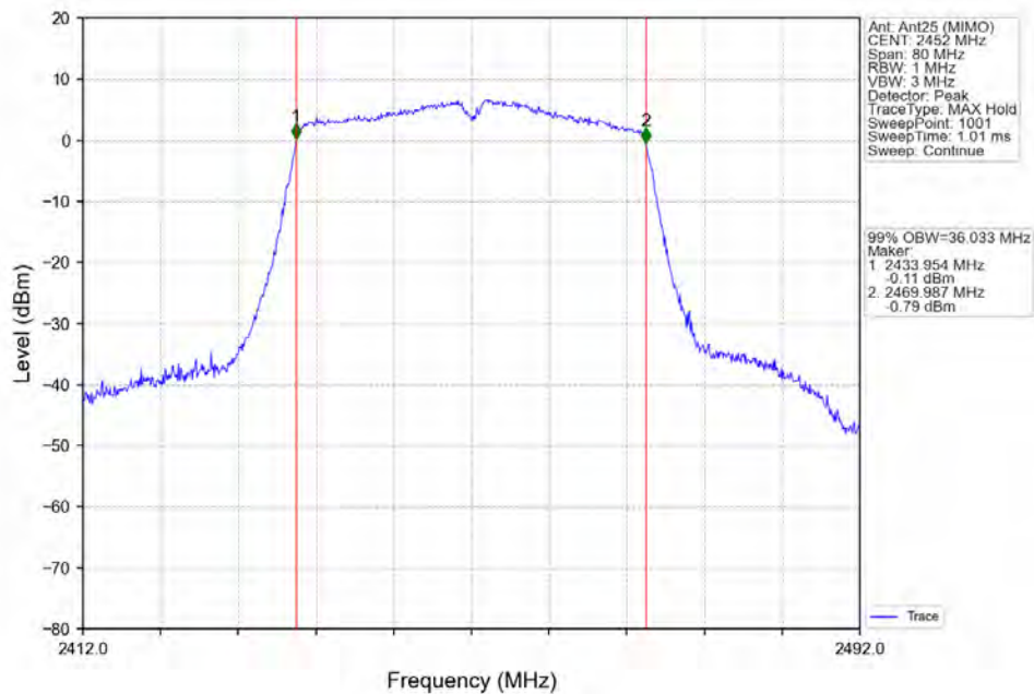
802.11ac(VHT40) HCH 2452MHz Ant25 (MIMO) NTNV
