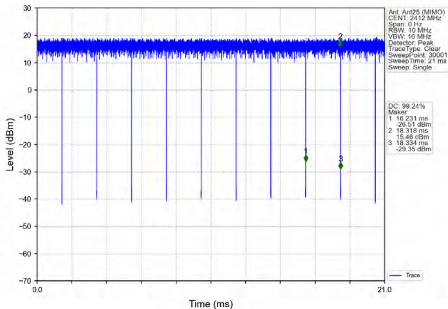
802.11g_LCH_2412MHz_Ant25 (MIMO)_NTNV
