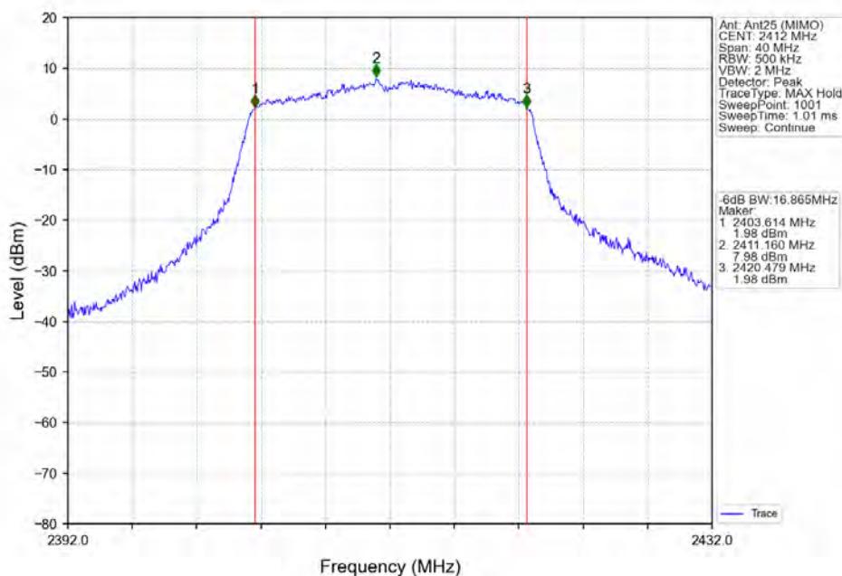
802.11n(HT20) LCH 2412MHz Ant25 (MIMO) NTV
