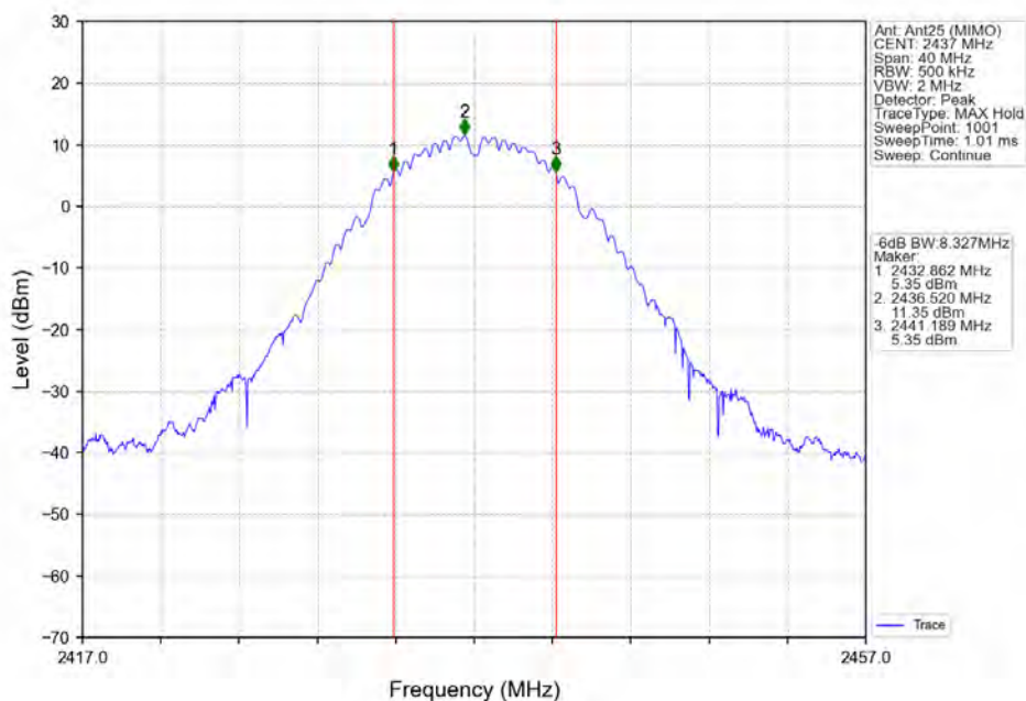
802.11b_MCH_2437MHz_Ant25 (MIMO)_NTNV
