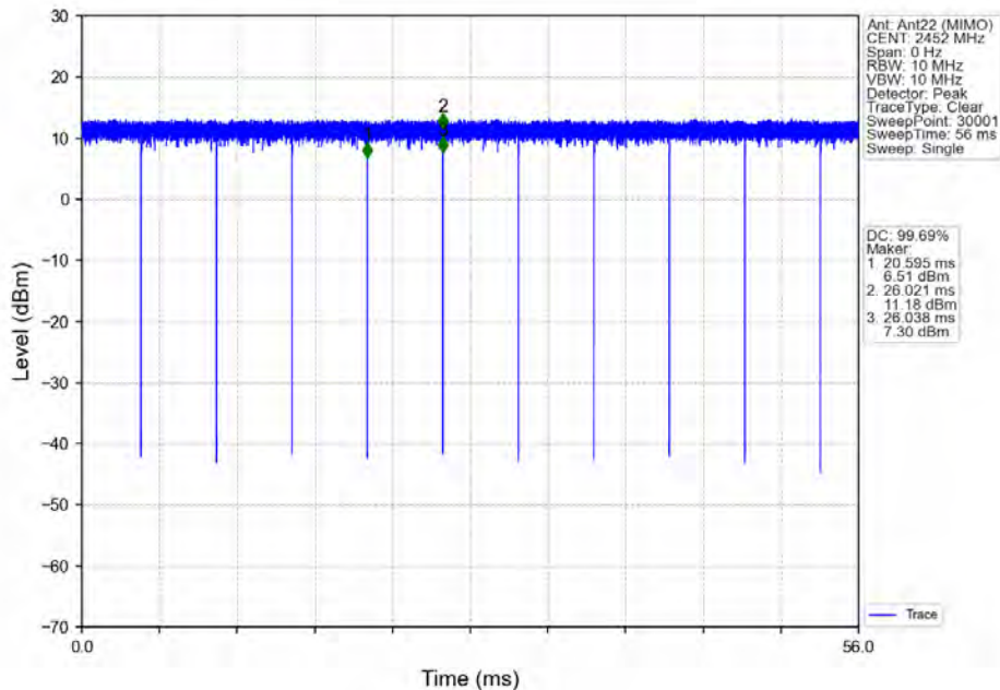
802.11n(HT40)_HCH_2452MHz_Ant22 (MIMO)_NTNV
