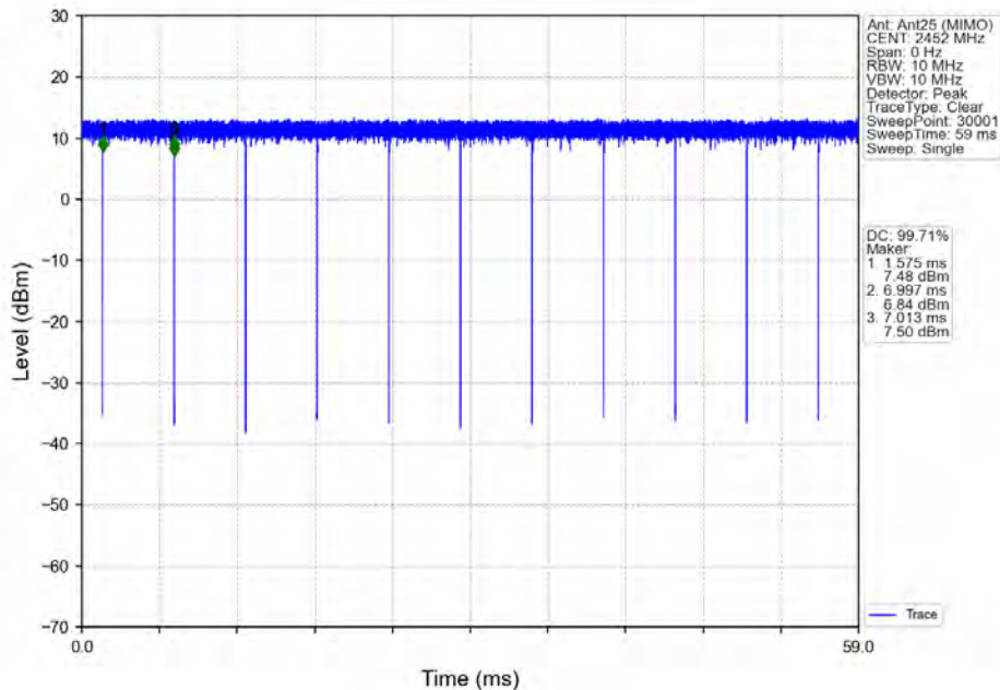
802.11n(HT40)_HCH_2452MHz_Ant25 (MIMO)_NTNV
