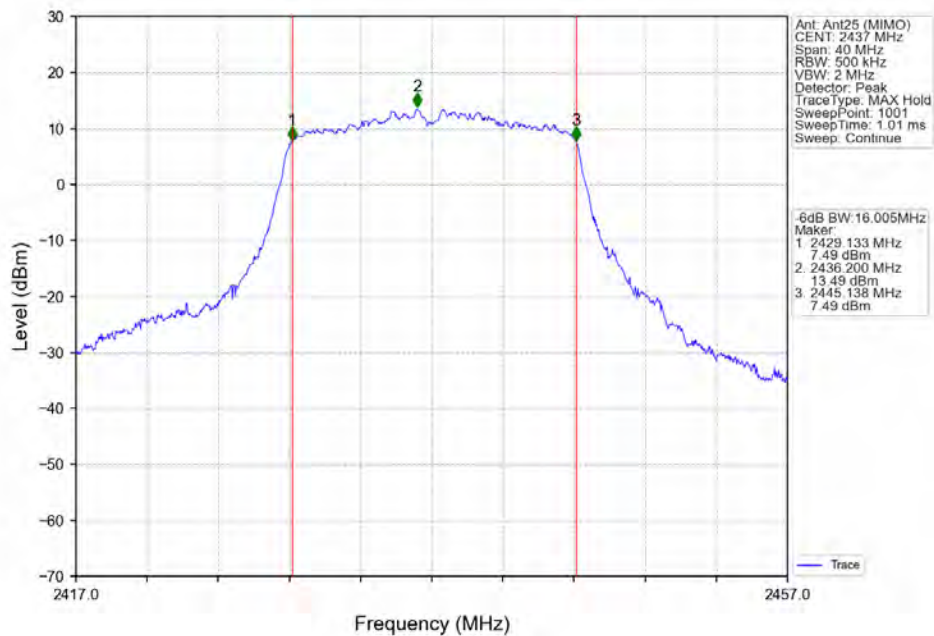
802.11g_MCH_2437MHz_Ant25 (MIMO)_NTNV
