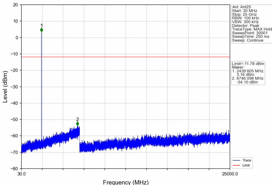
2M_MCH_2440MHz_Ant25_NTNV
