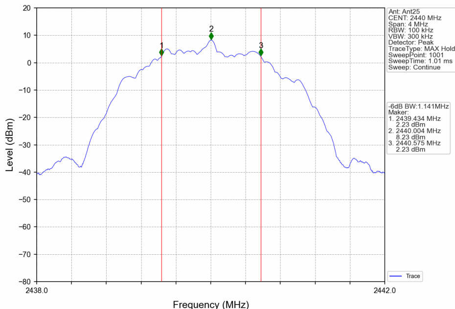
2M_MCH_2440MHz_Ant25_NTNV
