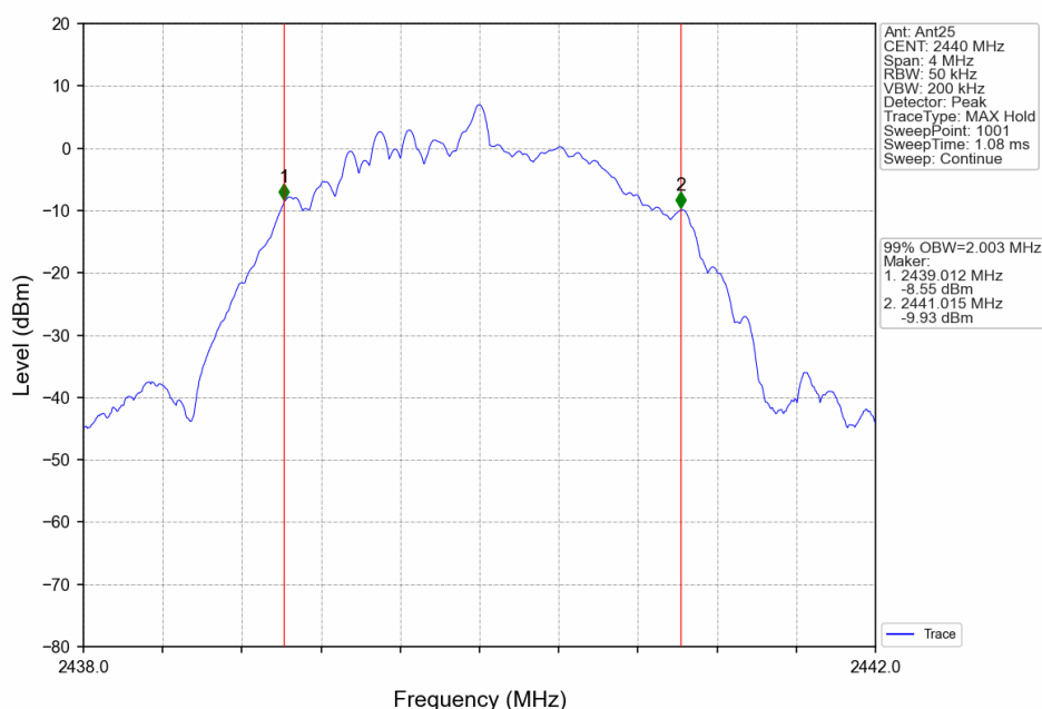
2M_MCH_2440MHz_Ant25_NTNV
