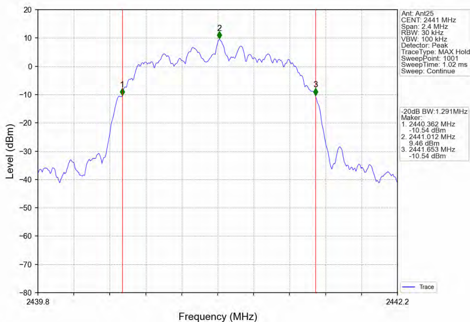
Pi/4DQPSK 2DH5 MCH 2441MHz Ant25 NTN
