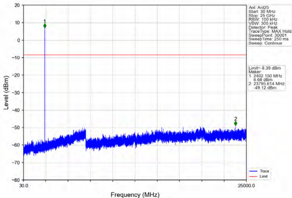
Pi/4DQPSK 2DH5 LCH 2402MHz Ant25 NTNV
